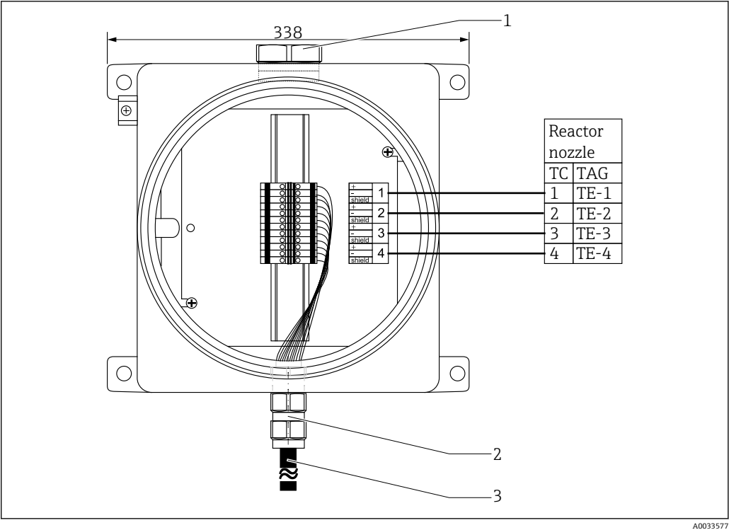
1 接线实例：TS901（带 4 个符合 IEC 60584 标准的 K 型热电偶铠装芯子（单支））通过屏蔽延长电缆连接安装在接线箱中的接线端子
