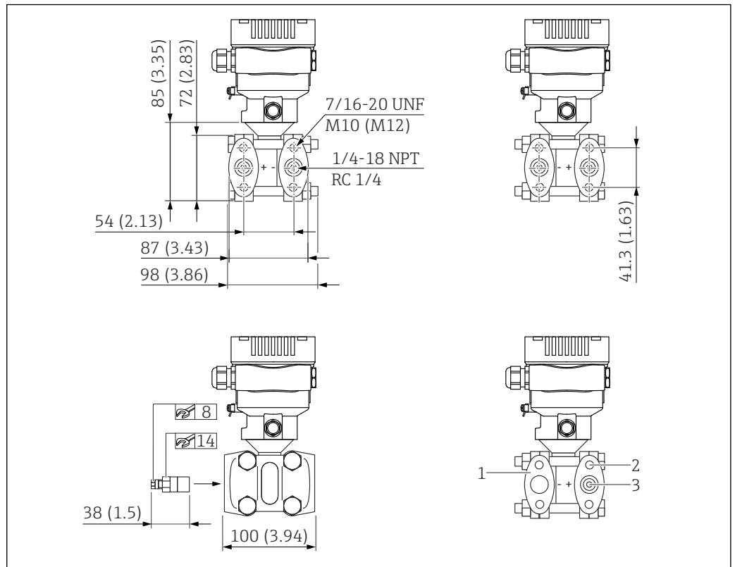
5 Vue de face, vue du côté gauche, vue du côté droit. Unité de mesure mm (in)
