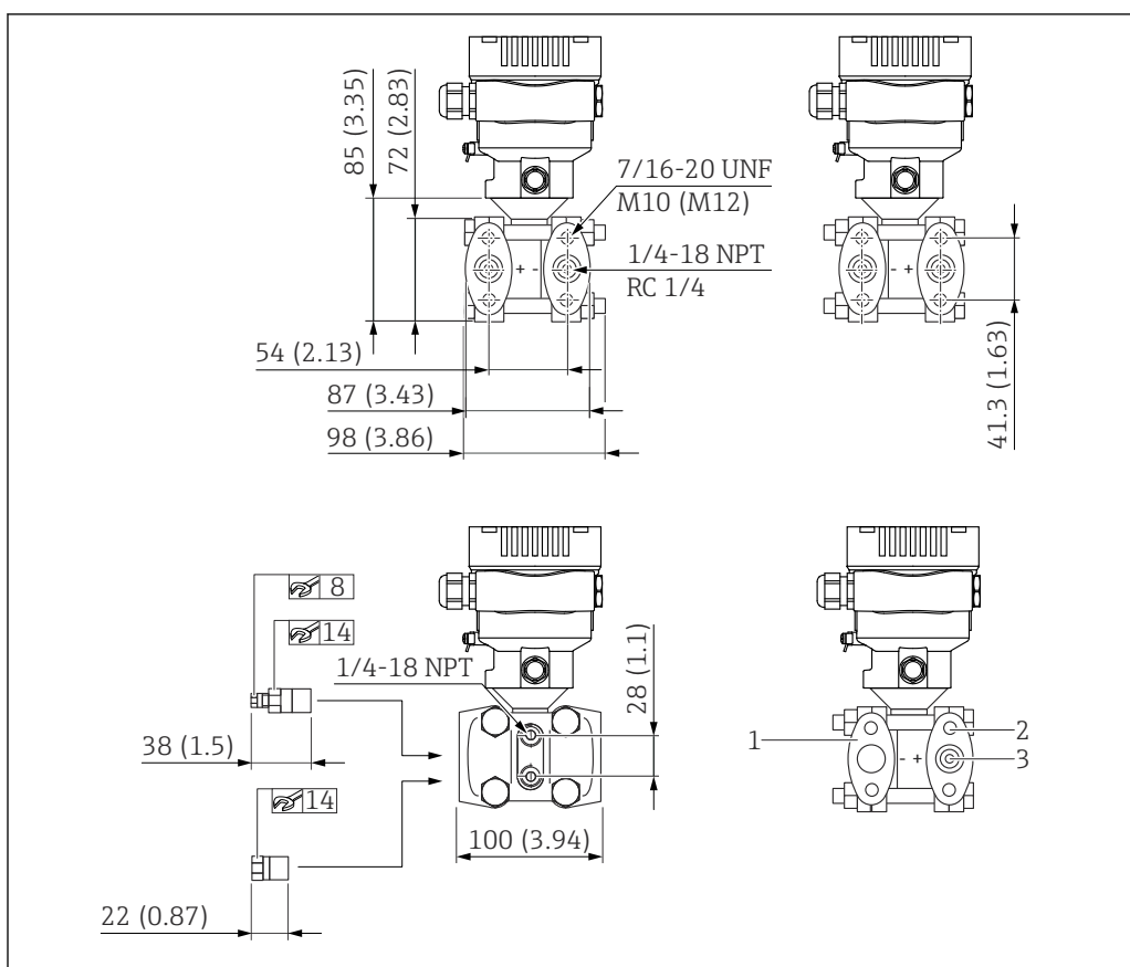
6 Vue de face, vue du côté gauche, vue du côté droit. Les écrous se trouvent toujours du côté négatif. Unité de mesure mm (in)
