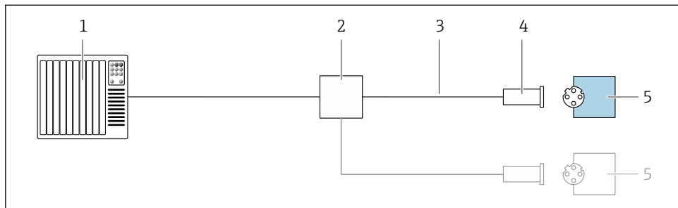
図 16 EtherNet/IP の接続例
