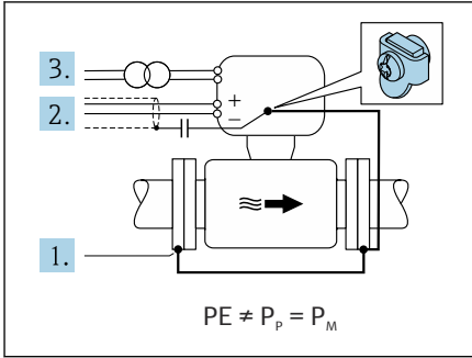
図 12 Promag L, W
