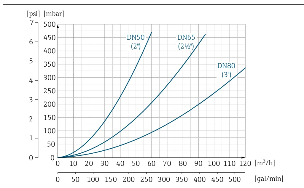
28 Perte de charge DN 50 à 80 (2 to 3") pour caractéristique de commande "Construction", option C "Bride fixe, tube de mesure rétréci", sections d'entrée/de sortie 0 x DN"
