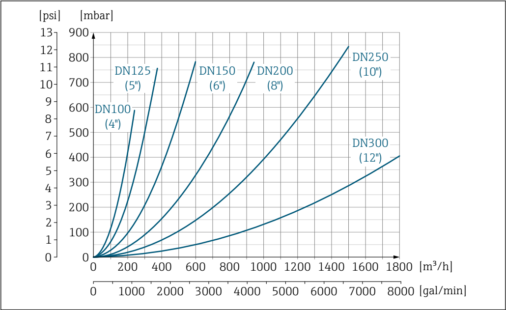
29 Perte de charge DN 100 à 300 (4 to 12") pour caractéristique de commande "Construction", option C "Bride fixe, tube de mesure rétréci", sections d'entrée/de sortie 0 x DN"
