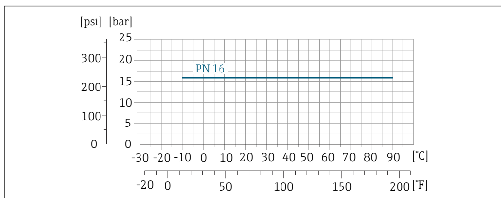
26 Matériau du raccord process : acier au carbone
