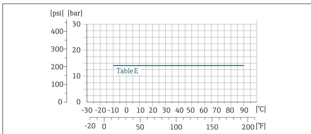
25 Matériau du raccord process : acier au carbone
