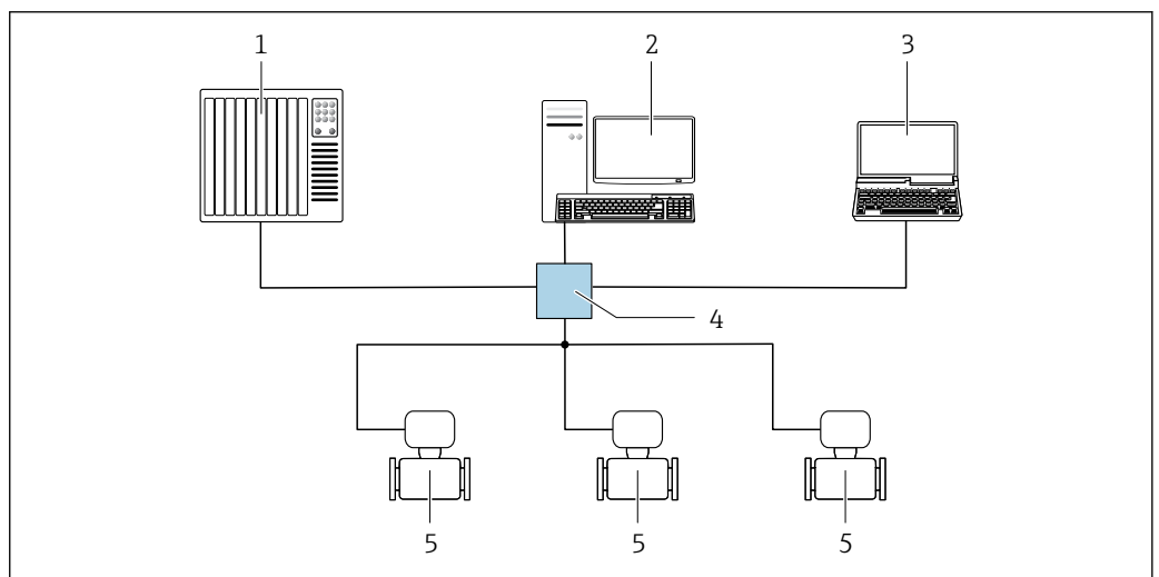
35 Options pour la configuration à distance via le réseau EtherNet/IP : topologie en étoile
