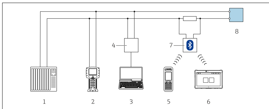
32 Possibilités de configuration à distance via protocole HART
