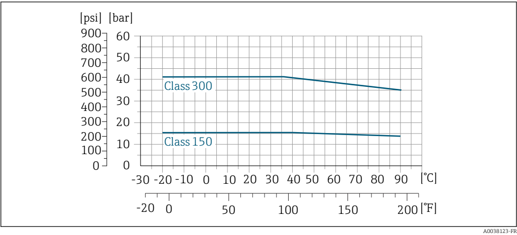
21 Matériau du raccord process : inox
