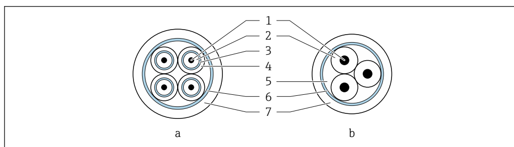
13 Section de câble
