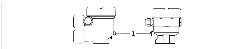
1 Zemnicí svorka pro připojení vedení ochranného pospojování
