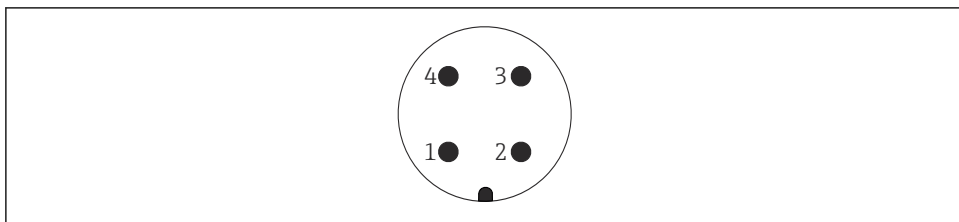
18 Zástrčka M12, přiřazení pinů
