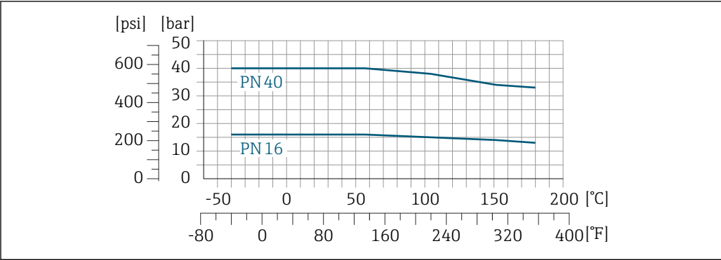
39 Avec matériau de bride 1.4404/F316L/F316
