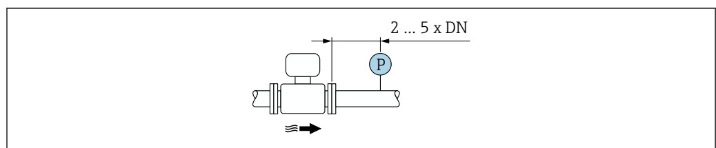
13 Montage d'un point de mesure de pression (P = transmetteur de pression)
