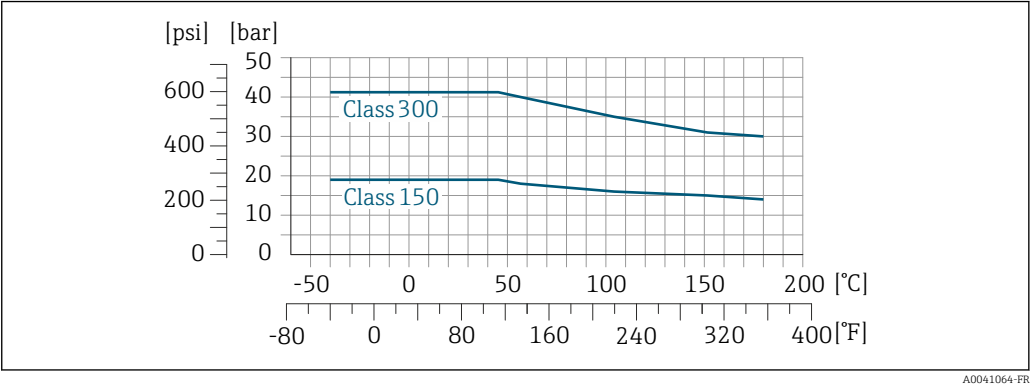
41 Avec matériau de bride 1.4404/F316L/F316
