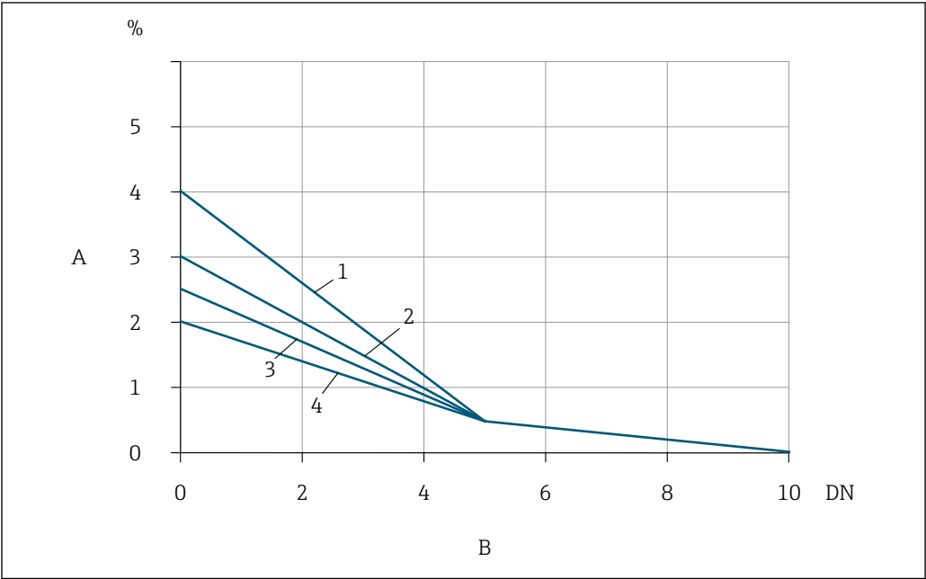
12 Error medido adicional que cabe esperar con acondicionadores de flujo en función del tipo de perturbación y del tramo recto de entrada A Error medido adicional (%) B Tramos rectos de entrada (DN) 1 2 codos de 90°, tridimensional 2 Expansión 3 2 codos de 90° 4 Reducción o codo de 90°
