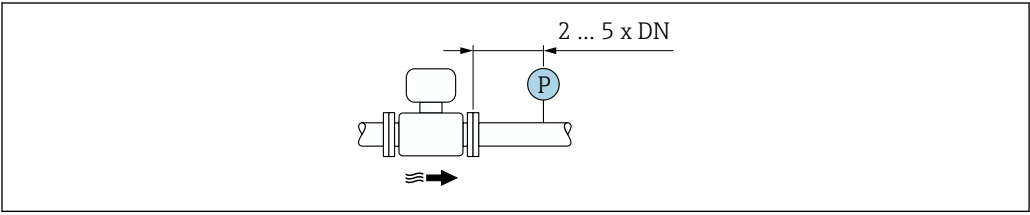
13 Instalación de un punto de medición de presión (P = transmisor de presión)
