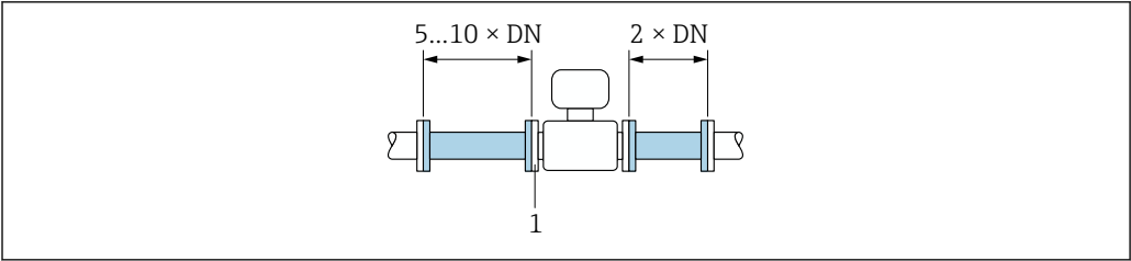
11 Tramos rectos de entrada y salida recomendados en caso de uso de una placa acondicionadora de caudal 1 Acondicionador de caudal
