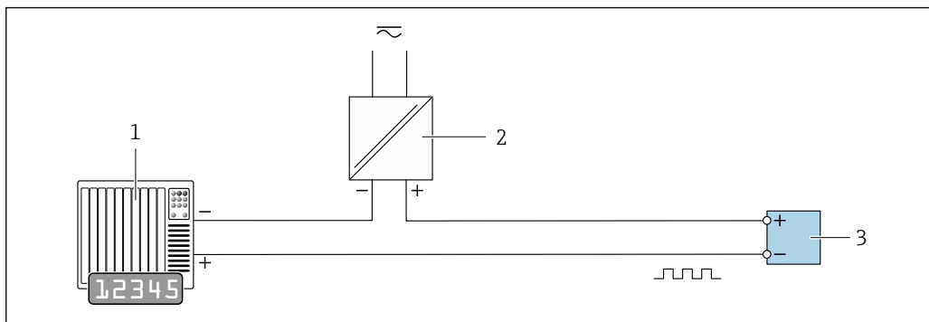
图 12 接线示例：脉冲/频率输出（无源信号）
