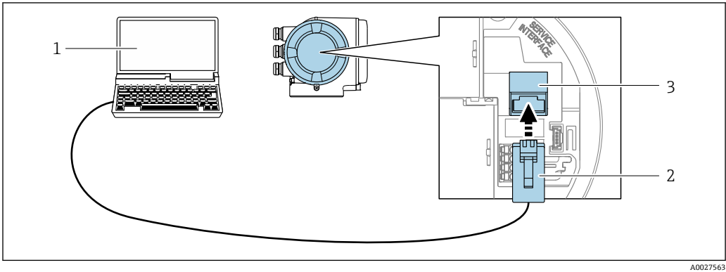
图 24 通过服务接口 (CDI-RJ45) 连接 1 计算机, 安装有网页浏览器 (例如 Microsoft Internet 浏览器、Microsoft Edge), 用于访问设备内置以 太网服务器; 或安装有 FieldCare、DeviceCare 调试软件, 支持 COM DTM“CDI 通信 TCP/IP”或 Modbus DTM 2 标准以太网连接电缆, 带 RJ45 连接头 3 测量设备的服务接口 (CDI-RJ45), 内置以太网服务器访问接口
