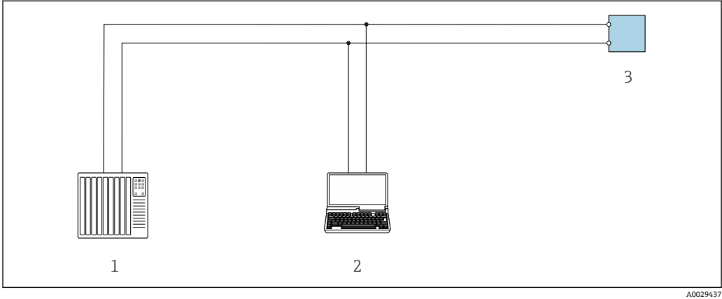
图 23 通过 Modbus-RS485 通信进行远程操作(有源信号) 1 控制系统(例如: PLC) 2 带 Web 浏览器的计算机(例如: Internet 浏览器), 用于访问内置设备 Web 服务器, 或安装有调试工具的计 算(例如: FieldCare、DeviceCare), 带 COM DTM “CDI 通信 TCP/IP”或 Modbus DTM 3 变送器
