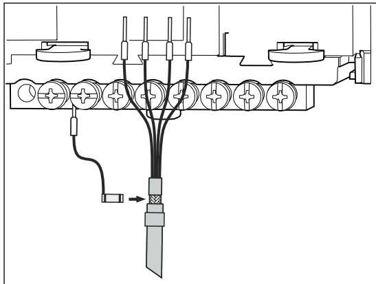
28 Conexión de tierra funcional
