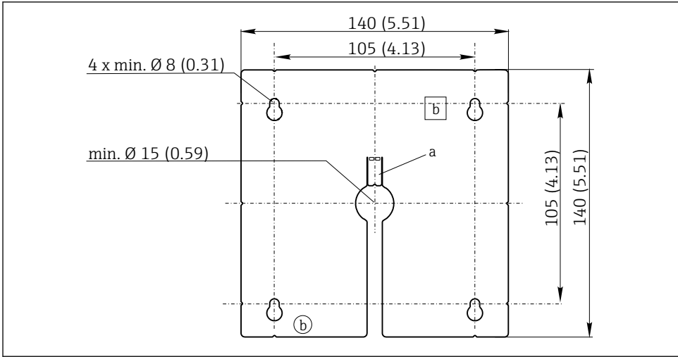
5 Placa de montaje para el indicador externo, dimensiones en mm (pulgadas)
