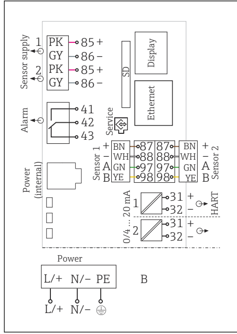
26 Diagrama de conexión completo con el ejemplo del BASE2-E y fuente de alimentación externa (B)
