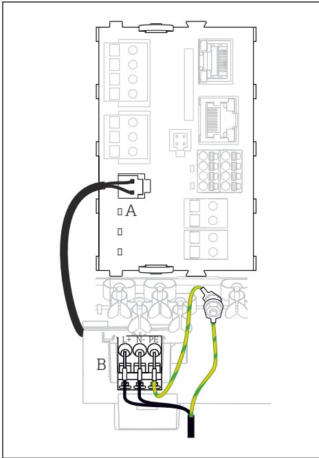
23 Conexión de la fuente de alimentación con el ejemplo del BASE2-E (equipo de campo)
