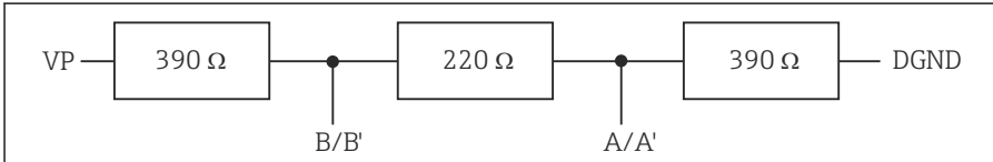
Fig. 59 Estructura del resistor de terminación interno
