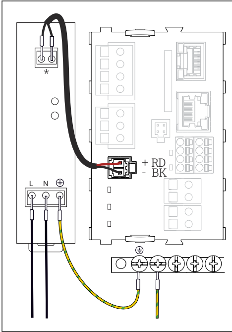
25 Conexión de la fuente de alimentación con el ejemplo del BASE2-E (equipo de armario)
