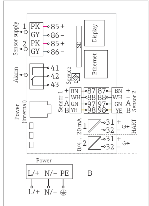
24 Diagrama de conexión completo con el ejemplo del BASE2-E y fuente de alimentación de expansión (B)
