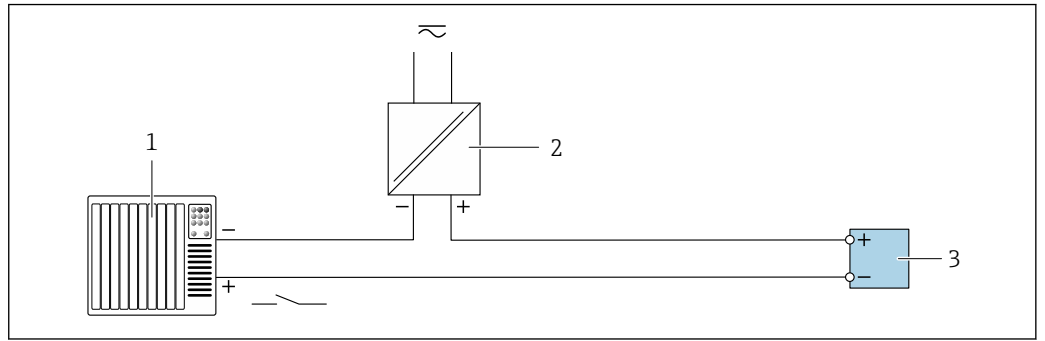
图 50 状态输入的连接示例
