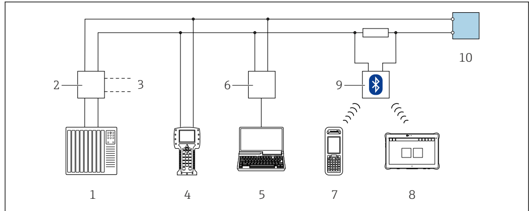
图 56 通过 HART 通信进行远程操作（无源信号）
