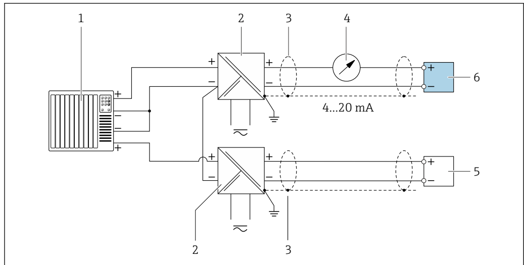
图 41 带公共终端的 HART 输入的连接实例 (无源)
