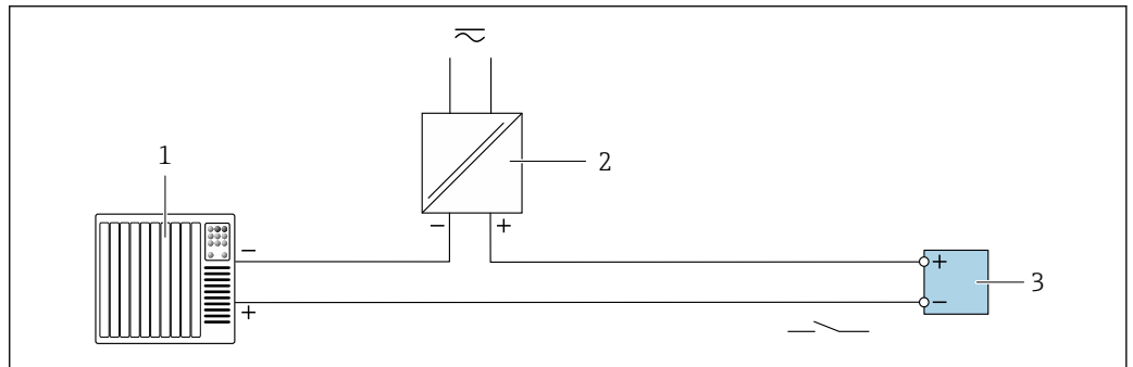
图 45 开关量输出(无源信号)的连接实例
