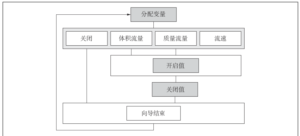
图 61 “设置”菜单中的“小流量切除”设置向导
