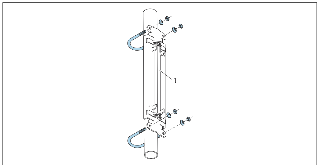
15 带 U 型螺丝的传感器安装支座
