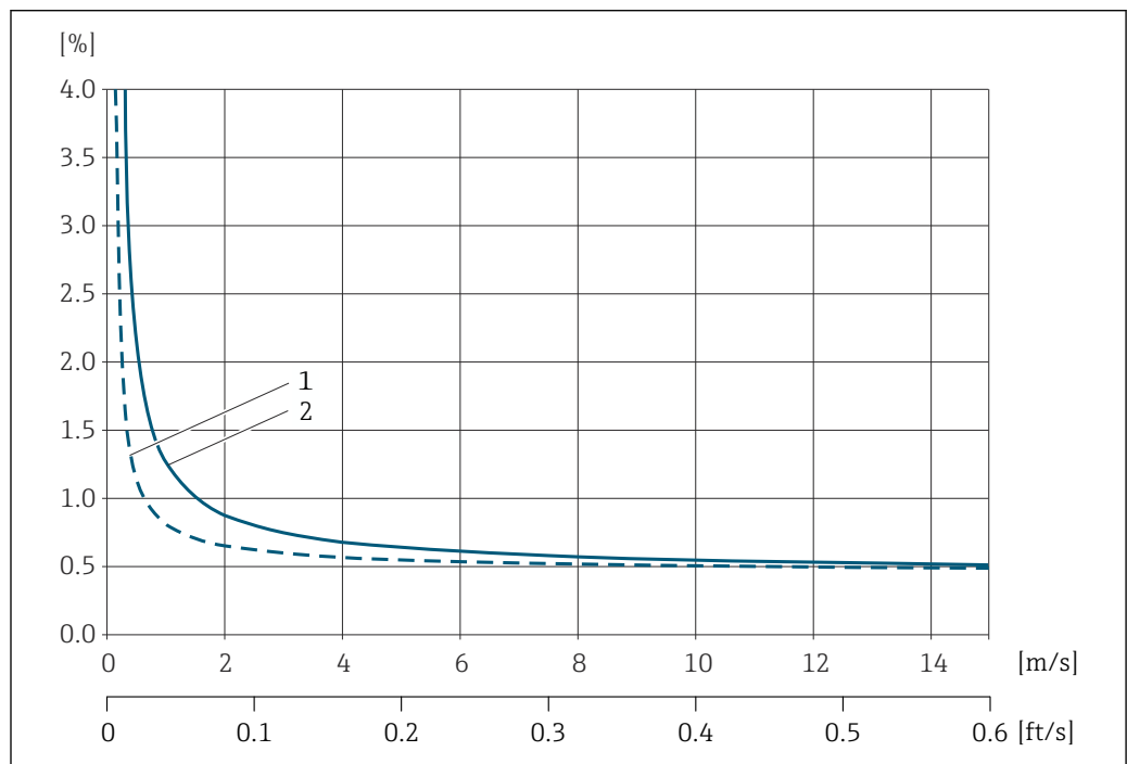
图 67 最大测量误差 (体积流量) (% o.r.) 的计算实例
