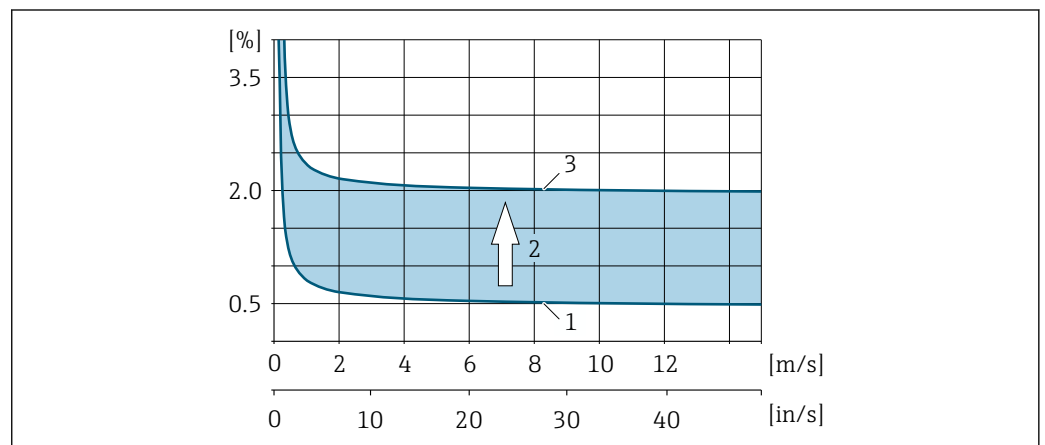
图 66 公称口径 DN > 200 (8") 的管道中的测量误差实例
