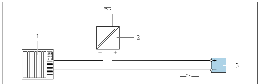
图 48 继电器输出的连接实例(无源)
