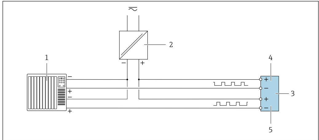
图 47 脉冲（相移）输出的连接实例（无源信号）
