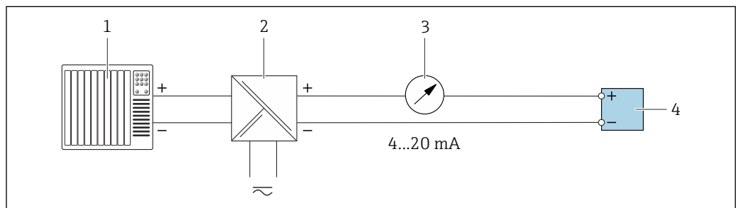
图 43 4...20 mA 电流输出 (无源) 的连接示例
