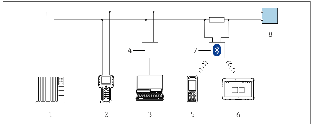
图 55 通过 HART 通信进行远程操作（有源信号）
