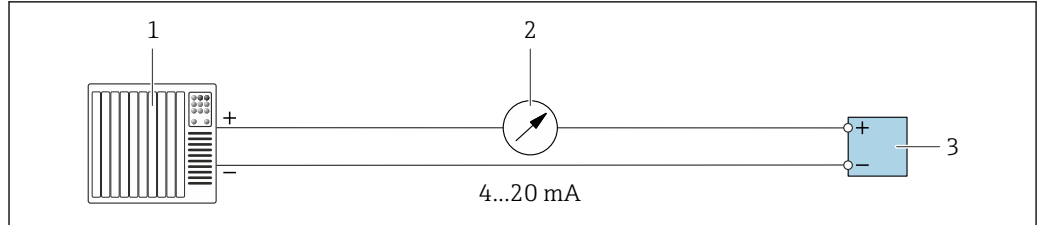
图 42 4...20 mA 有源电流输出的连接示例
