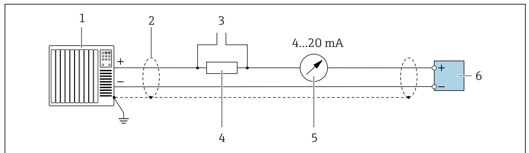
图 39 接线示例：4...20 mA HART 电流输出（有源信号）
