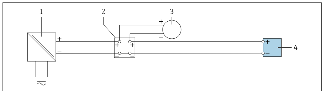
图 49 4...20 mA 电流输入的连接示例
