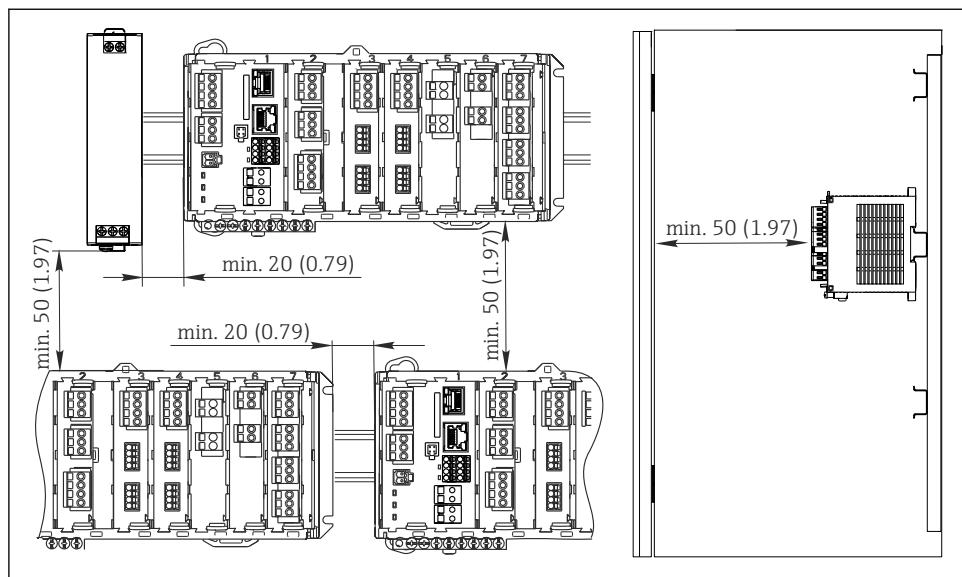
3 Dégagement minimum en mm (in)
