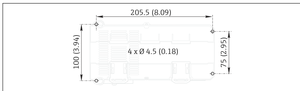
4 Gabarit de perçage pour montage mural en mm (in)
