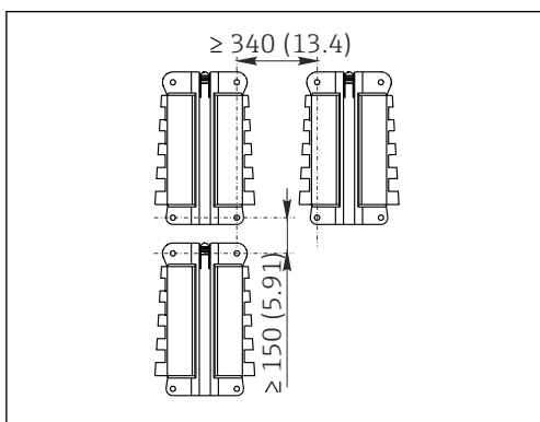
12 Dégagement de montage en mm (in)
