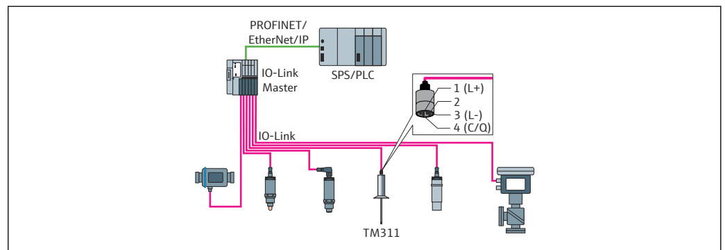
図 1 IO-Link 通信モードの M12 接続
