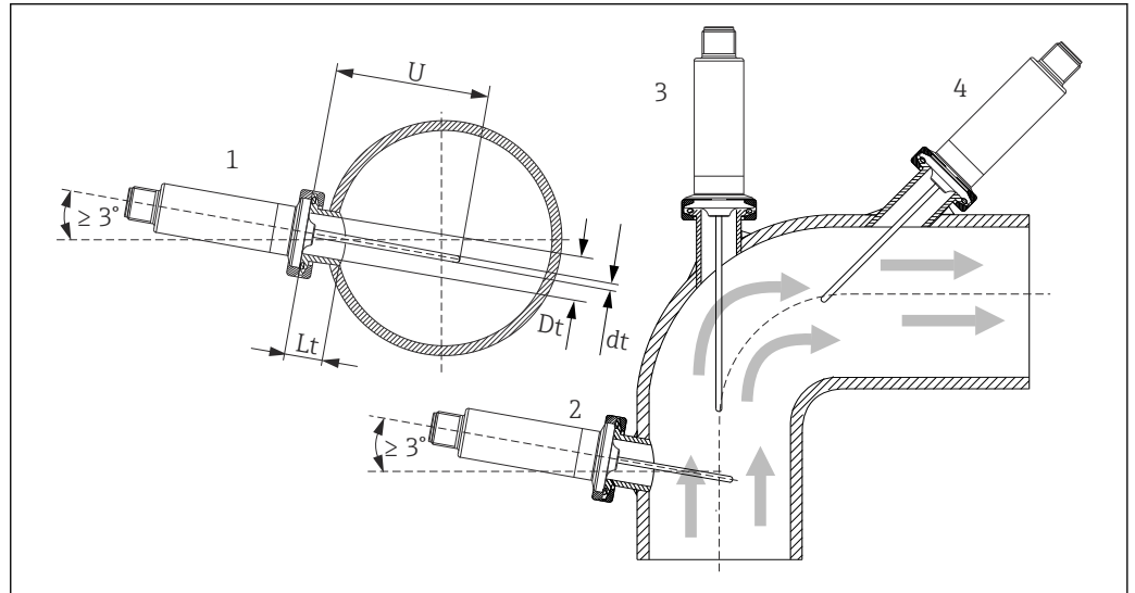
図 6 設置例
