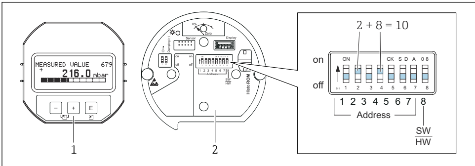
3 Fig. 8: setarea adresei dispozitivului prin intermediul comutatoarelor de tip DIP switch
