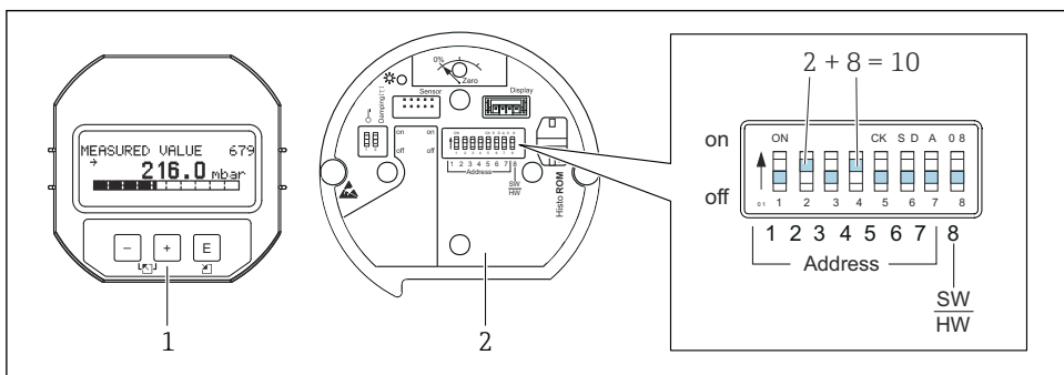
Fig. 8: Impostazione dell'indirizzo dei dispositivi tramite microinterruttori DIP
