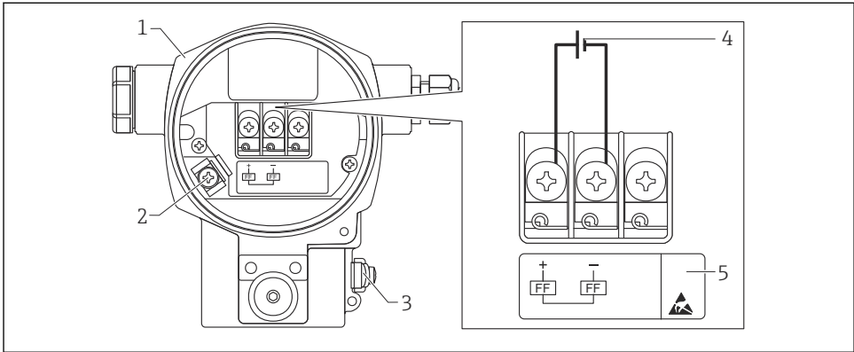
1 FOUNDATION Fieldbus elektromos csatlakoztatás
