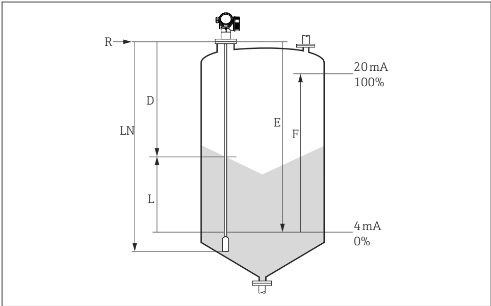
19 Konfigurációs paraméterek ömlesztett szilárd anyagokban történő szintméréshez
