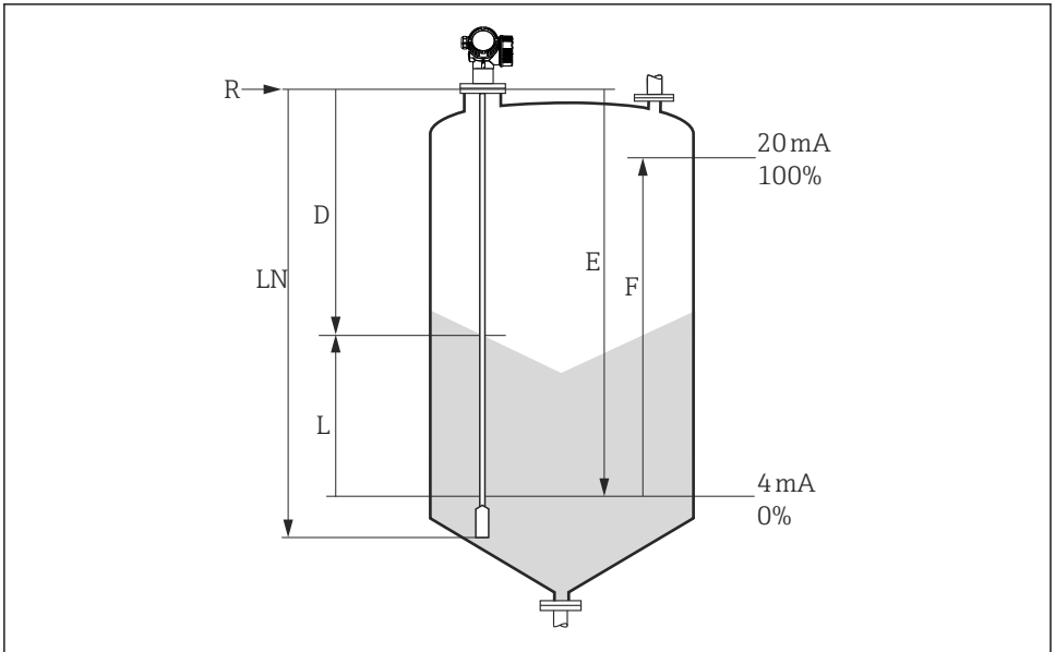
19 Parametri de configurare pentru măsurarea nivelului de substanțe solide în vrac
