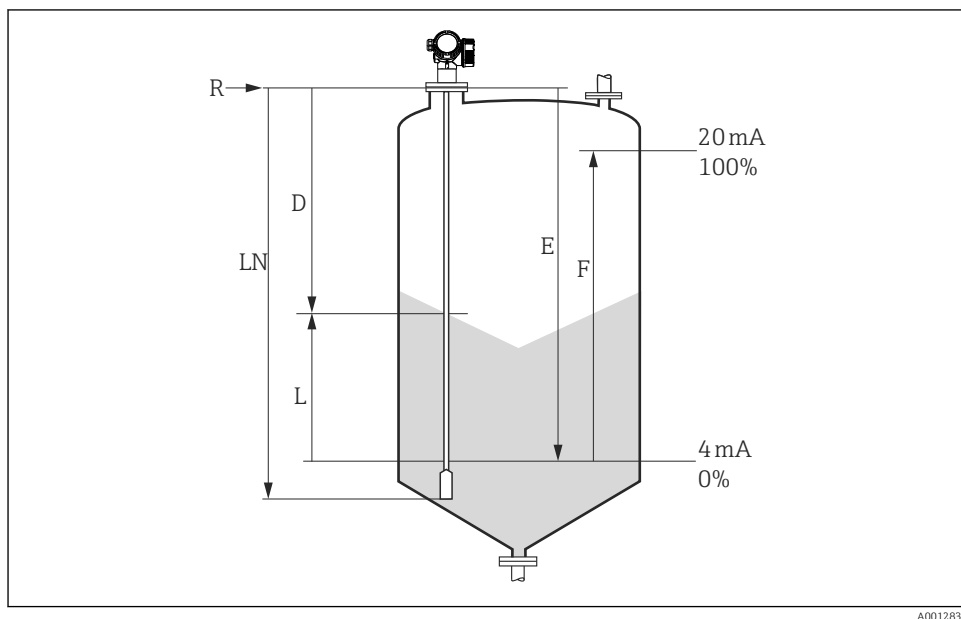
19 Paramètres de configuration pour la mesure de niveau dans les solides en vrac
