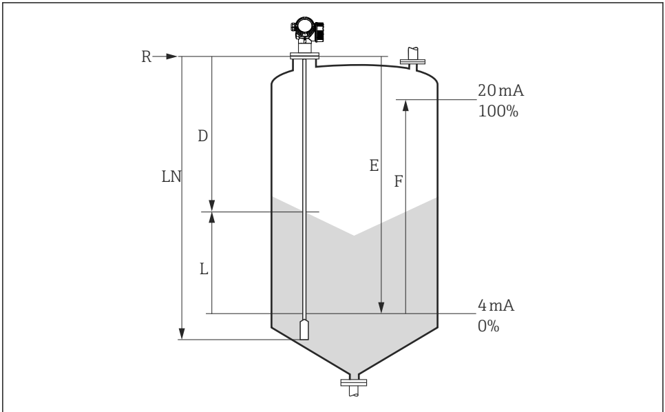
19 Parametry konfiguracyjne pomiaru poziomu materiałów sypkich
