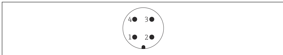
12 Rozmieszczenie styków w gnieździe przyłączeniowym M12
