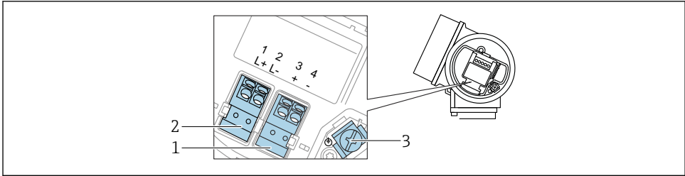
図 8 端子の割当て、4線式：4~20 mA HART (10.4~48 V DC )
