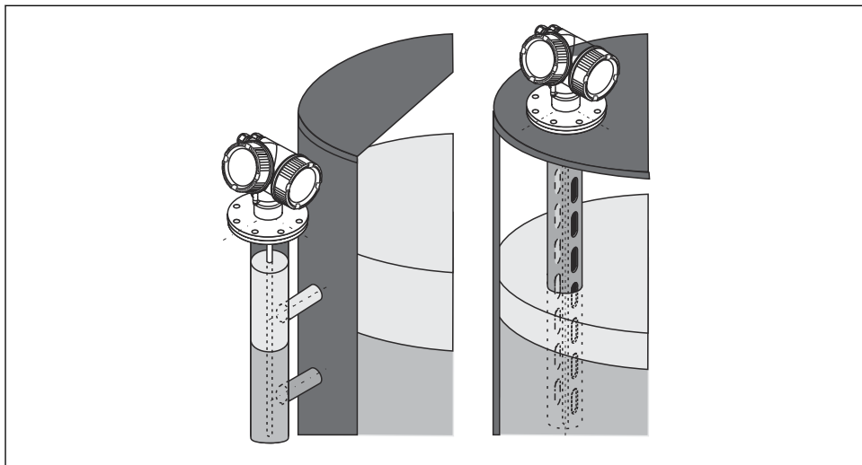
1 Montážní poloha u Levelflex FMP55
