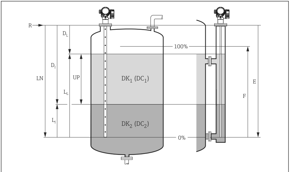
10 Konfigurointiparametrit rajapintamittaukseen
