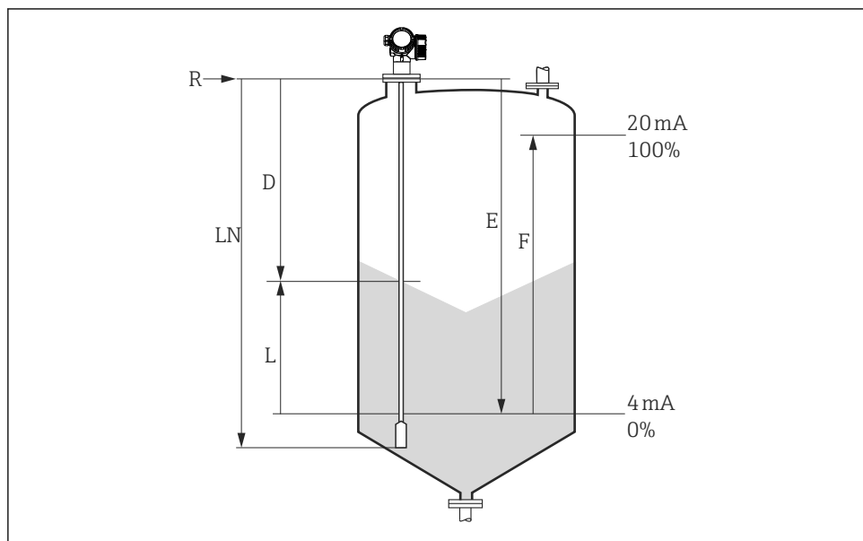
11 Konfiguracijski parametri za meritve nivoja sipkih snovi
