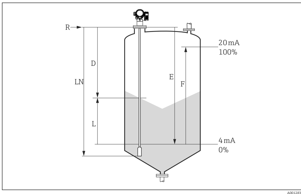
11 Konfigurációs paraméterek ömlesztett szilárd anyagokban történő szintméréshez
