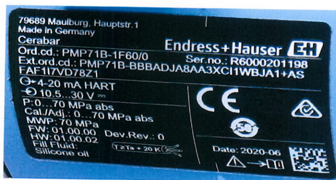
Рисунок 2. Маркировка преобразователей
