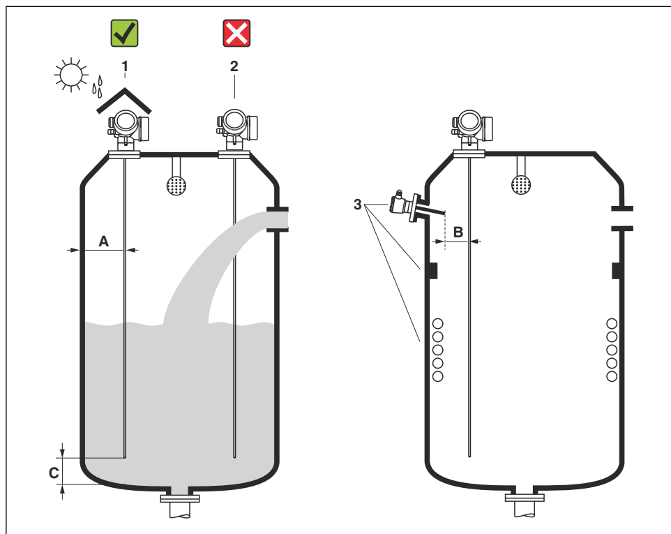
1 Condiciones de instalación para Levelflex
