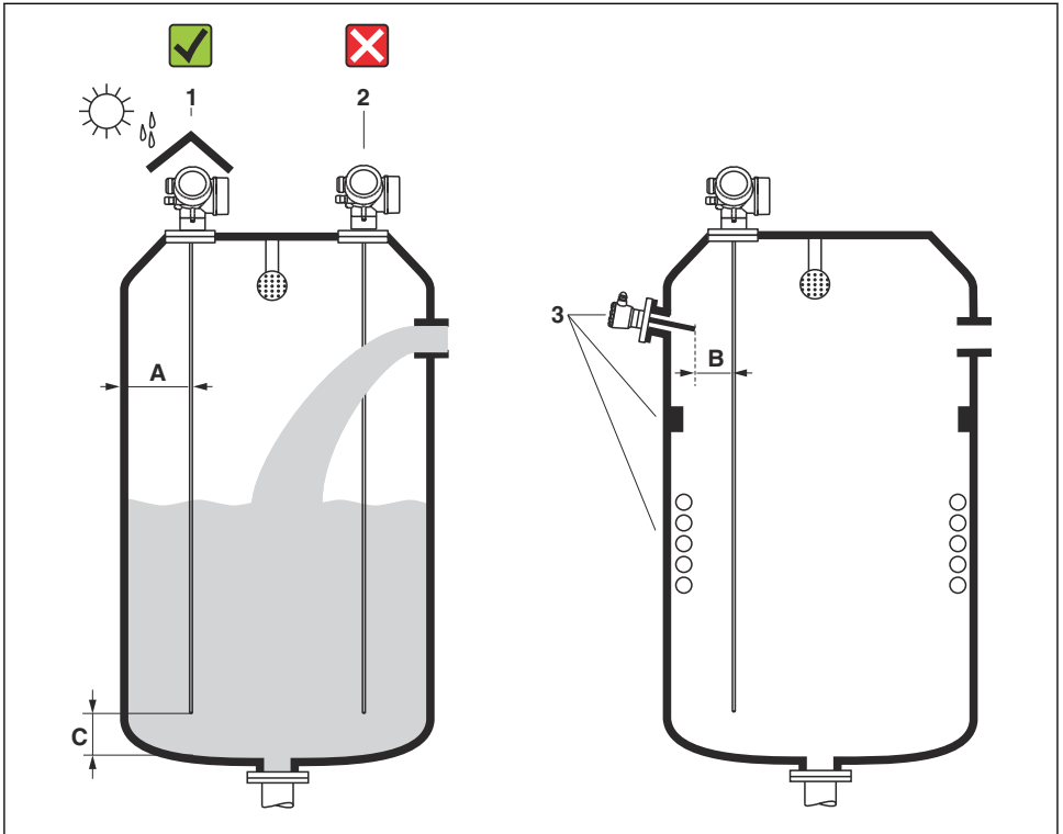
1 Condiții de instalare pentru Levelflex
