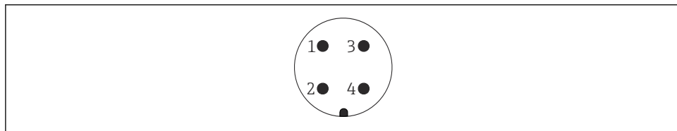
4 Affectation des broches du connecteur 7/8"
