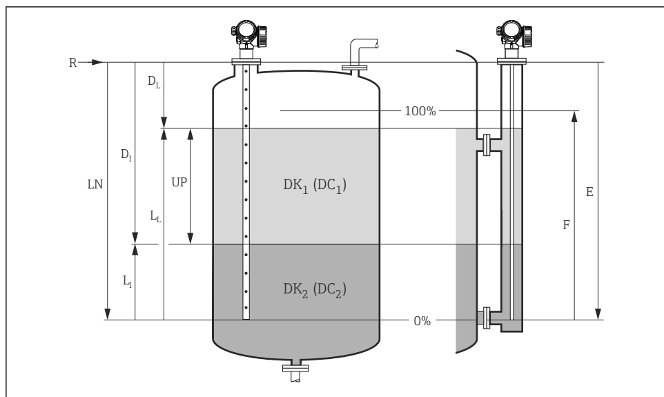
10 Paramètres de configuration pour la mesure d'interface
