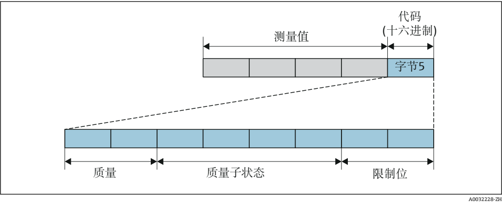
图 25 编码字节结构
