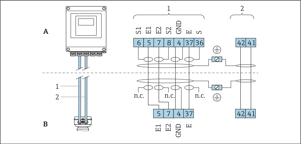
图 7 分体型仪表的接线端子分配
