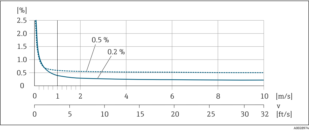
28 最大测量误差 (% o.r.)
