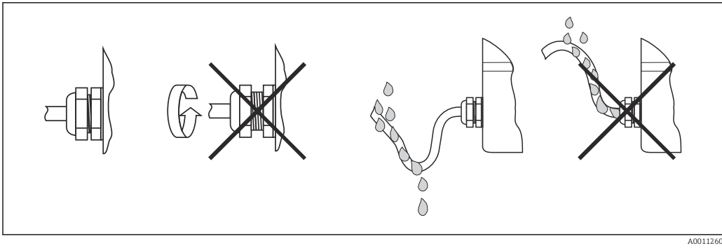
12 Anschlusshinweise zur Einhaltung der Schutzart IP
