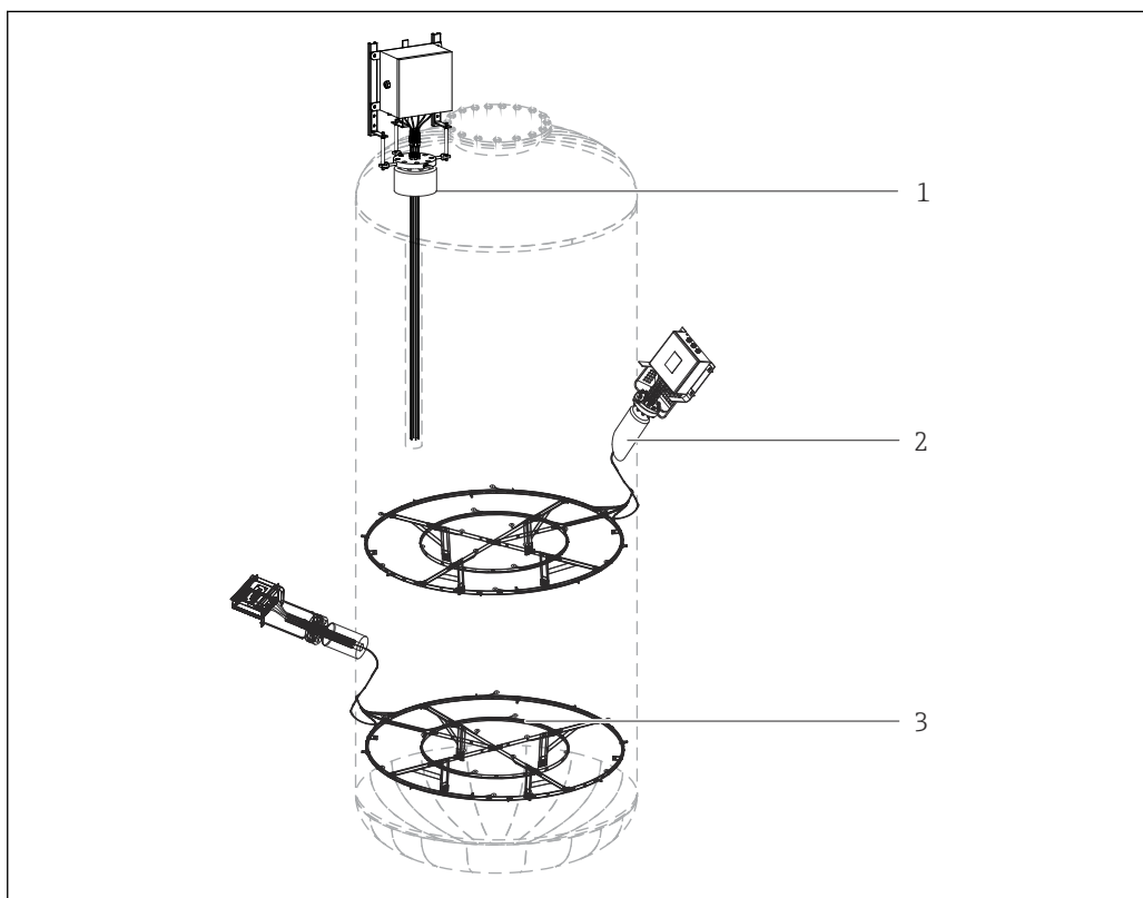
3 Einbaubeispiele – keine Beschränkungen hinsichtlich der Einbaulage
