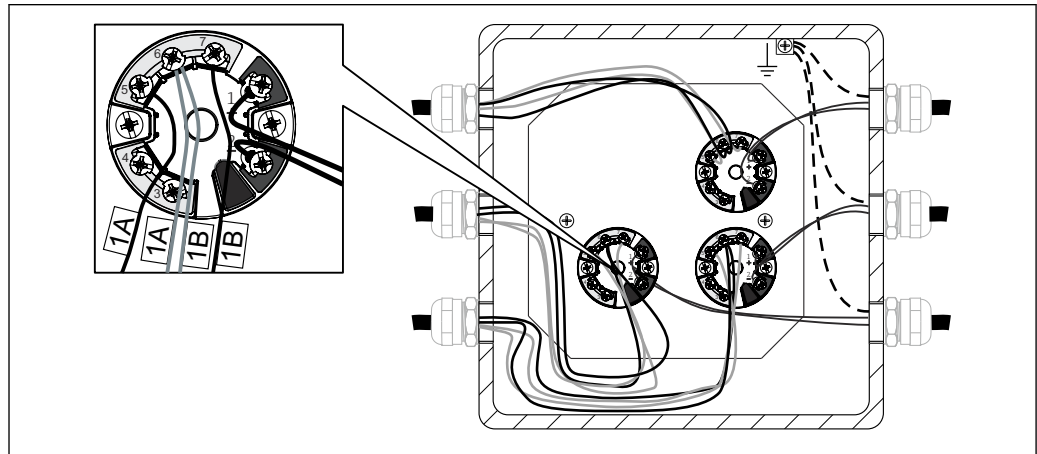
10 Montierter und verdrahteter Kopftransmitter. Beispiel für die interne Kennzeichnung der Sensorleitungen bei 2 Thermoelementen
