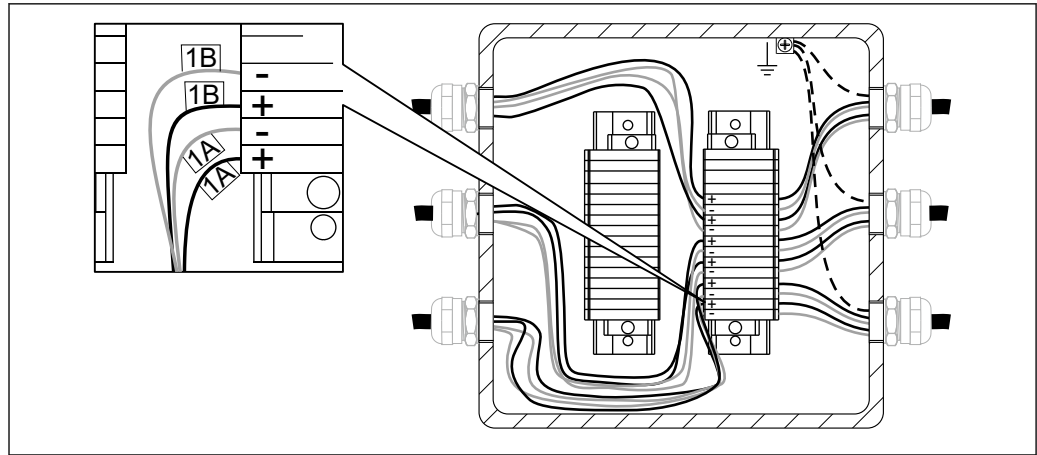
9 Direkte Verdrahtung auf dem montierten Anschlussklemmenblock. Beispiel für die interne Kennzeichnung der Sensorleitungen bei 2 Thermoelementsensoren in Messeinsatz 1.
