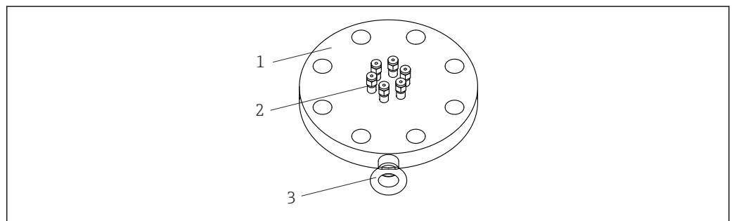
15 Flansch als Prozessanschluss
