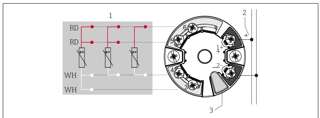
6 Im Anschlusskopf montierter Transmitter TMT7x oder TMT31 (ein Sensoreingang)
