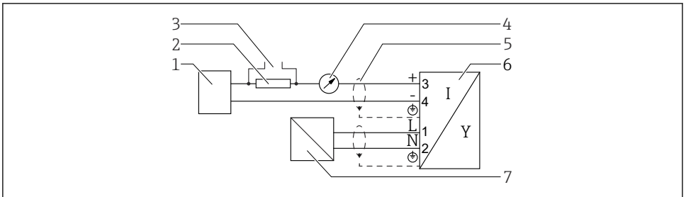
図 13 ブロック図、4線式：4~20 mA HART (90~253 V AC )
