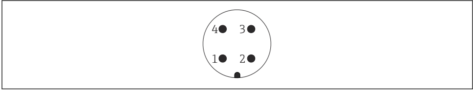
図 14 M12 プラグのピン割当て
