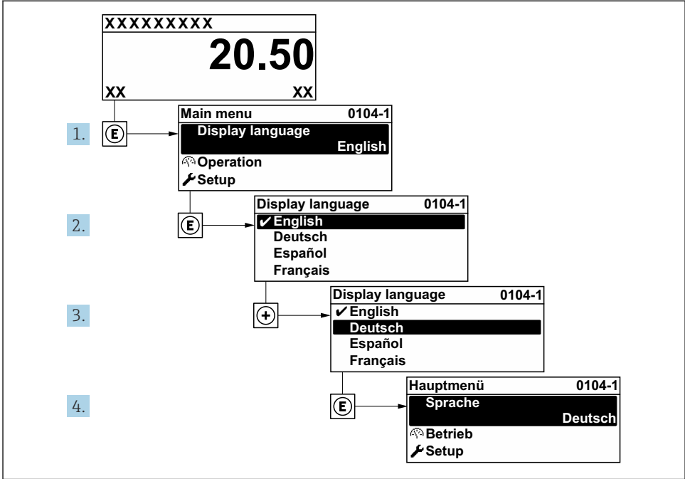
図 21 現場表示器の表示例
