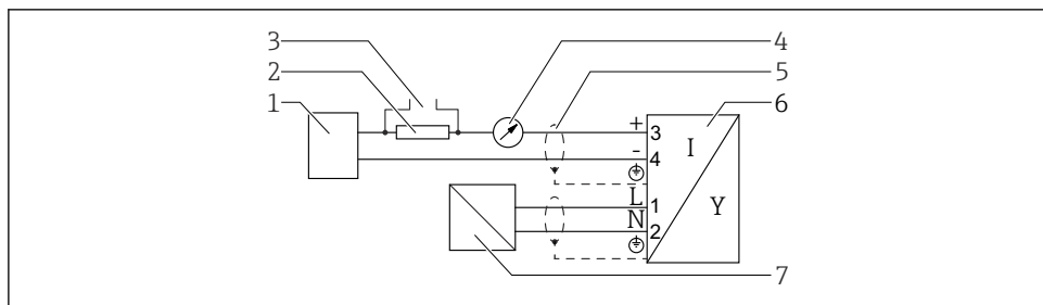
17 Diagrama de bloco, 4 fios: 4 para 20 mA HART (90 para 253 V AC )
