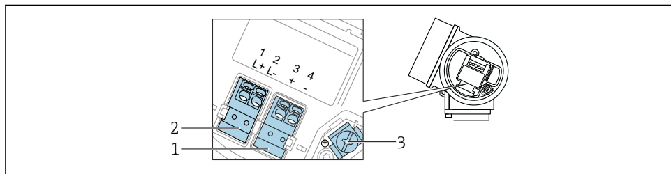
14 Esquema de ligação elétrica, 4 fios: 4 para 20 mA HART (10.4 para 48 V DC )
