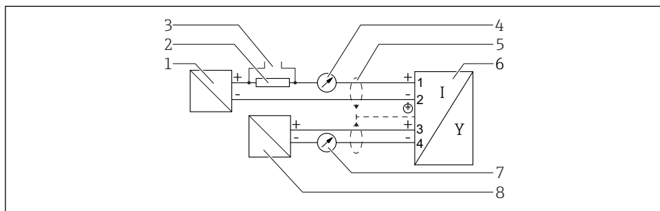
13 Diagrama de bloques, a 2 hilos: 4 ... 20 mA HART, 4 ... 20 mA
