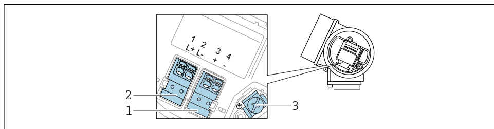
14 Asignación de terminales, a 4 hilos: 4 ... 20 mA HART (10,4 ... 48 V DC )
