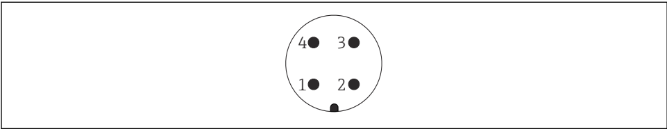
18 Asignación de pins del conector M12
