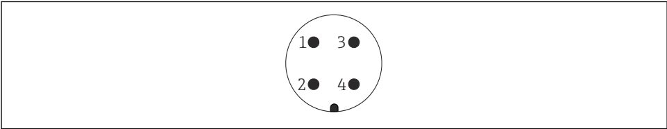
19 Asignación de pins del conector 7/8"
