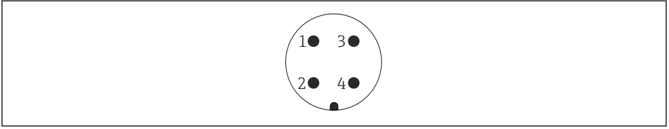
☐ 5 7/8" 플러그의 핀 할당
