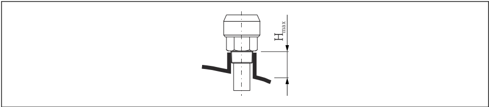
☞ 2 캡슐화된 혼 안테나의 노즐 높이(FMR50); H_{\max} = 60 \text{ mm} (2.36 in)
