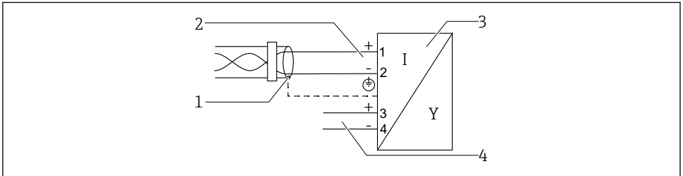
☐ 4 PROFIBUS PA / FOUNDATION Fieldbus 계통도
