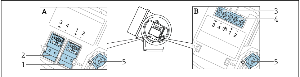
☐ 3 PROFIBUS PA / FOUNDATION Fieldbus 단자 할당
