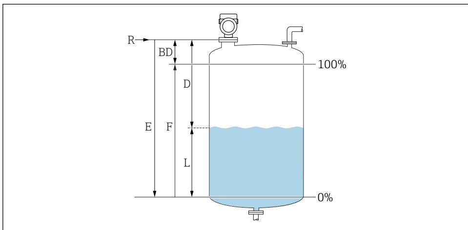
15 Parametri di configurazione per la misura di livello nei liquidi
