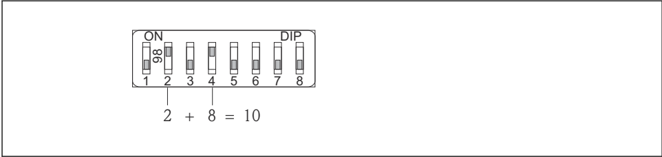
9 Példa hardveres címzésre: a 8-as kapcsoló „OFF” állásban van; az 1–7. kapcsolók határozzák meg a címet.
