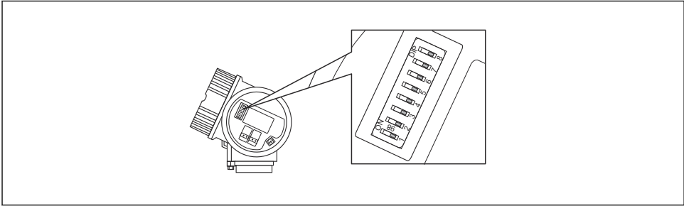
8 Címkapcsoló a csatlakozódobozban
