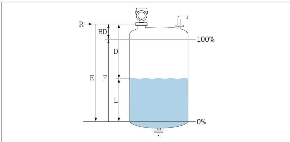
15 Параметры конфигурации для измерения уровня жидкости
