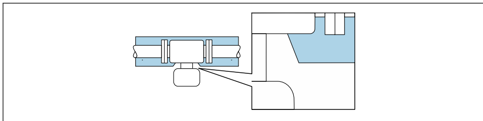
3 Tepelná izolace s volným prodlouženým krčkem
