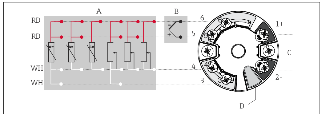
図 3 ヘッド組込型伝送器の端子接続の割当て
