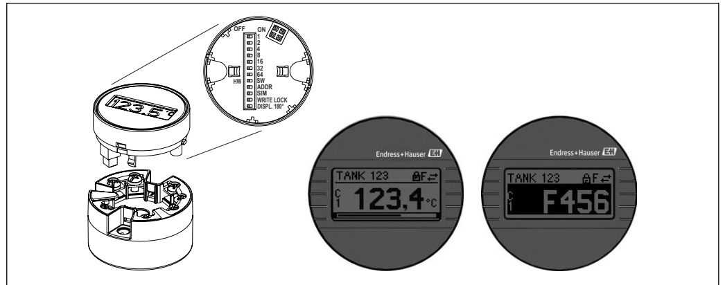
図 8 バーグラフインジケータ付き着脱式測定値ディスプレイ TID10 (オプション)
