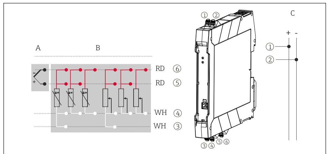
図 4 DIN レール伝送器の端子接続の割当て
