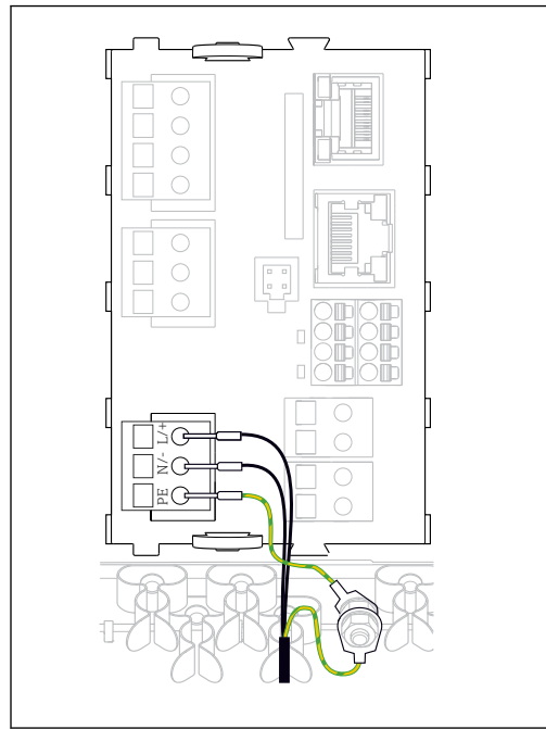
29 Conexión de la fuente de alimentación mediante el ejemplo del BASE2-H o -L
