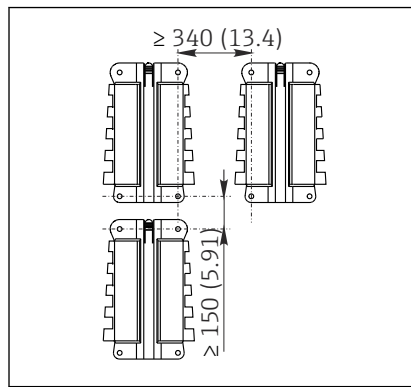
16 Espacio de instalación en mm (pulgadas)
