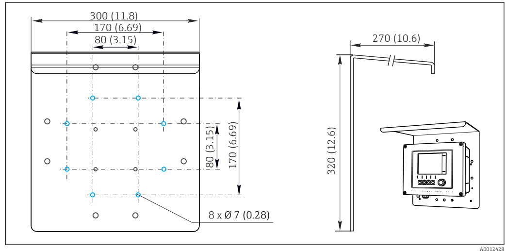
9 Dimensiones en mm (in)
