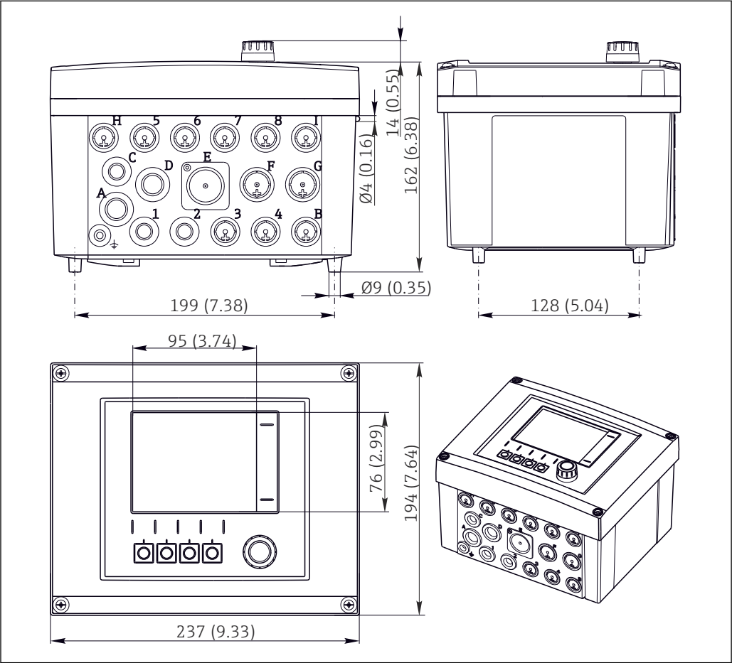
7 Medidas de la caja para montaje en campo en mm (in)
