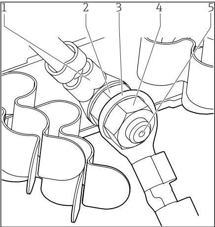
34 Conexión de tierra de protección o de puesta a tierra
