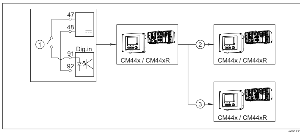
Fig. 79 Ejemplo de un control de limpieza central
