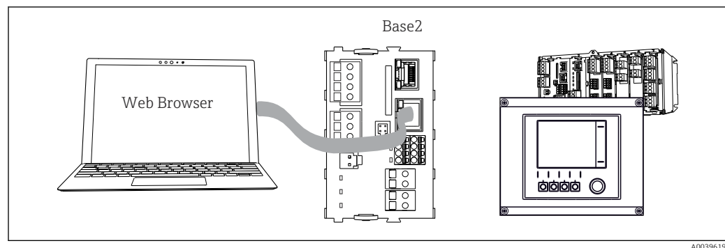
72 Servidor web/conexión Ethernet
