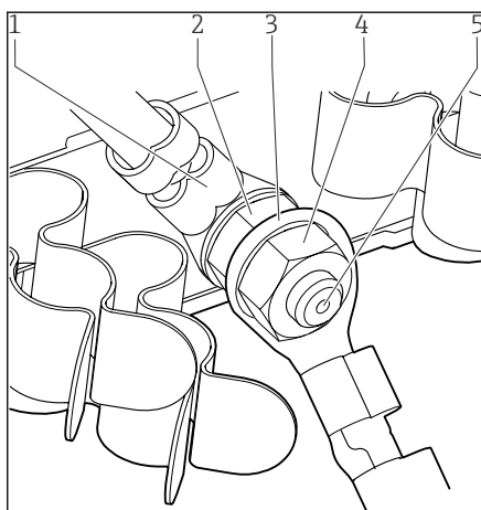
31 Conexión de tierra de protección o de puesta a tierra
