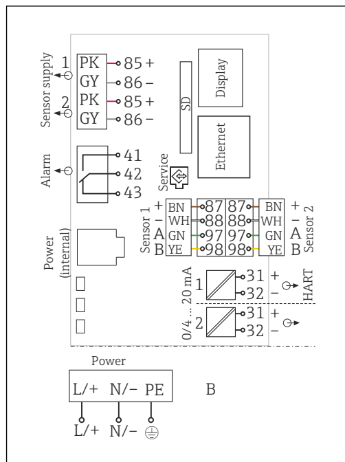
33 Diagrama de conexión completo con el ejemplo del BASE2-E y fuente de alimentación de expansión (B)
