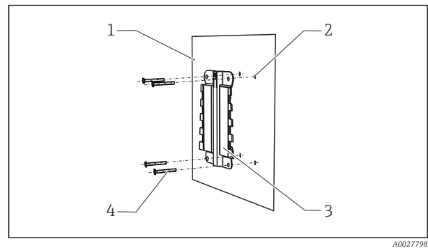
17 Montaje en pared
