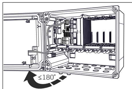
24 Abra la tapa que cubre la pantalla, ángulo máx. de apertura 180° (depende del lugar de montaje)
