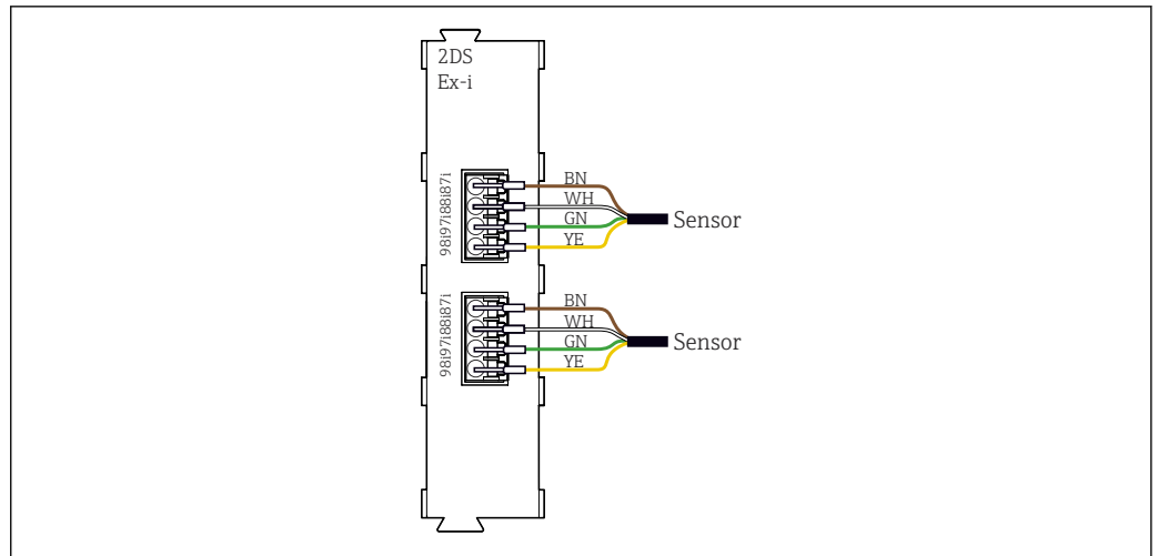
40 Sensores sin tensión de alimentación adicional en el módulo de comunicación del sensor de tipo 2DS Ex-i
