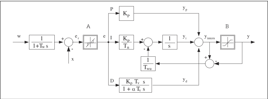
86 Diagrama de bloques de la estructura del controlador
