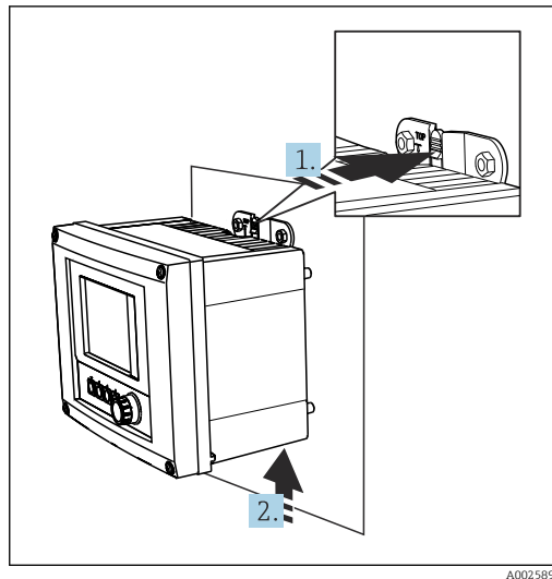
20 Desmontaje
