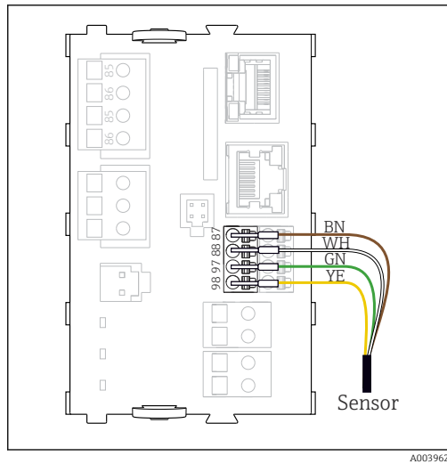
35 sensores sin fuente de alimentación adicional
