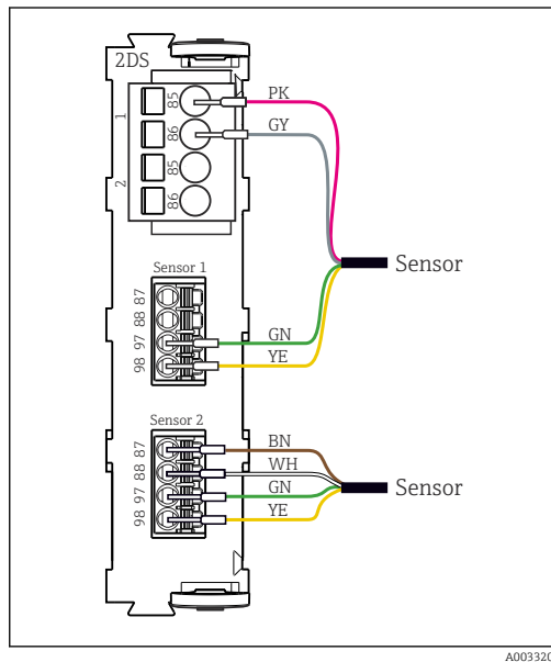
37 Sensores con y sin tensión de alimentación adicional en el módulo del sensor 2DS
