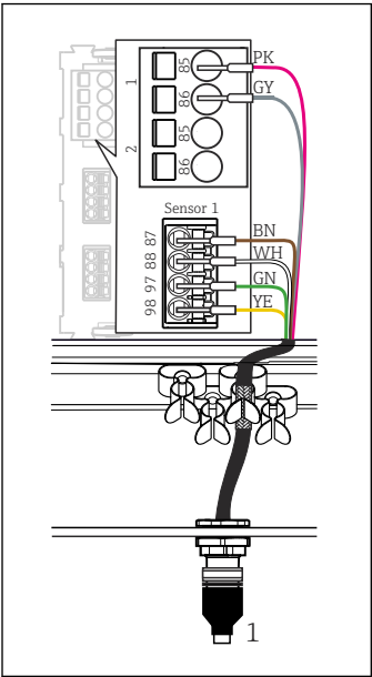
38 Conexión M12 (p. ej., en el módulo del sensor) 1 Cable de sensor con conector M12
