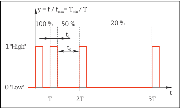
77 Aplicación típica: bomba dosificadora
