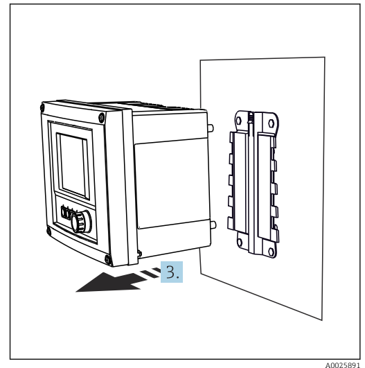
21 Desmontaje
