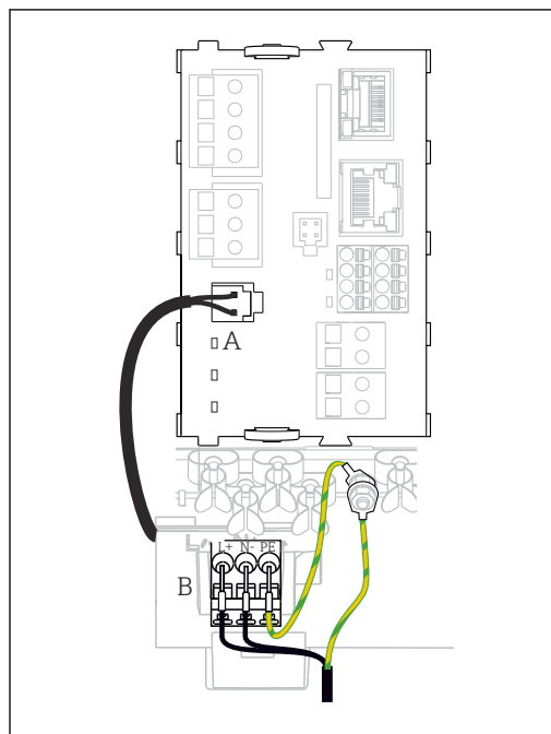
32 Conexión de la fuente de alimentación con el ejemplo del BASE2-E
