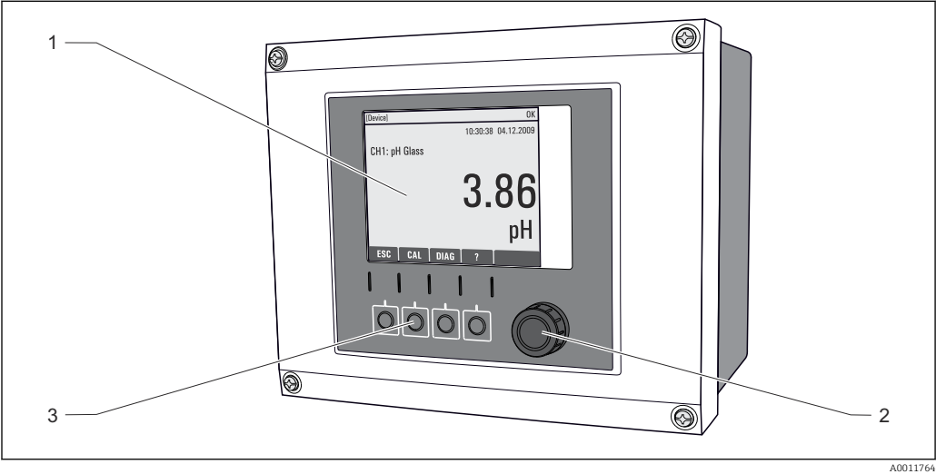
75 Visión general del funcionamiento 1 Indicador (con fondo rojo para el estado de alarma) 2 Navegador (funciones pulsar/retener y jog/shuttle) 3 Teclas de configuración rápida (su función depende del menú)
