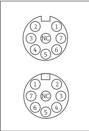
39 Asignación M12, superior: conector hembra; inferior: conector (vista superior en cada caso) 1 PK (rosa) (24 V) 2 GY (gris) (tierra 24 V) 3 BN (marrón) (3 V) 4 WH (blanco) (tierra 3 V) 5 GN (verde) (Memosens) 6 YE (amarillo) (Memosens) 7, No conectado NC
