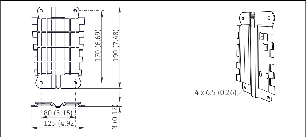
8 Placa de montaje. Unidad física: mm (in)
