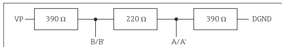
68 Estructura de la terminación interna
