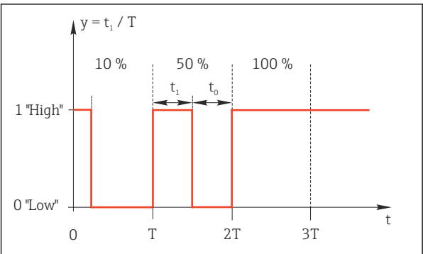
76 Aplicaciones típicas: válvula solenoide
