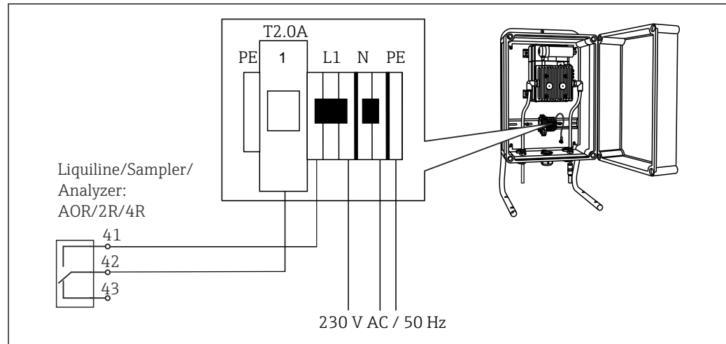
53 Conexión de la unidad de limpieza para CAS40D
