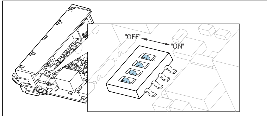
67 Microinterruptor de terminación interna
