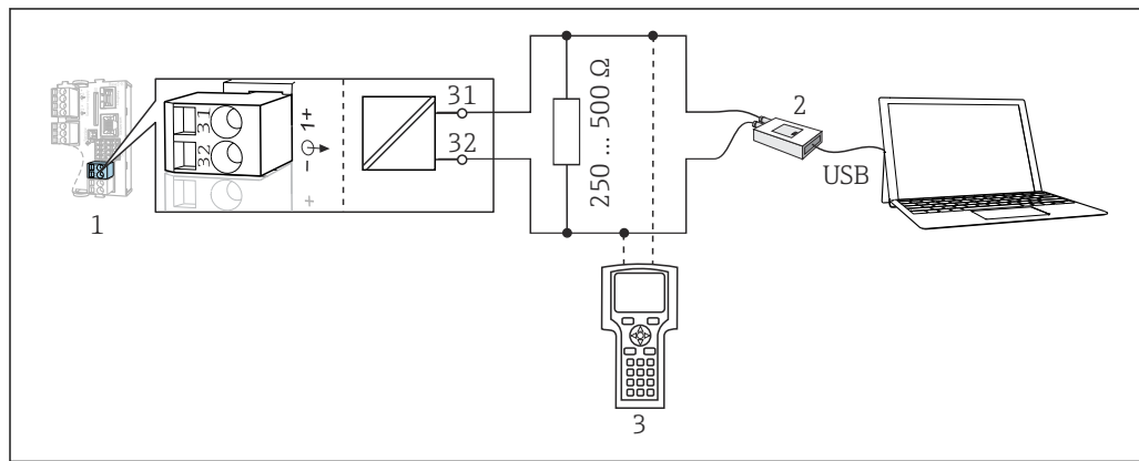
Fig. 22 Mediante módem HART
