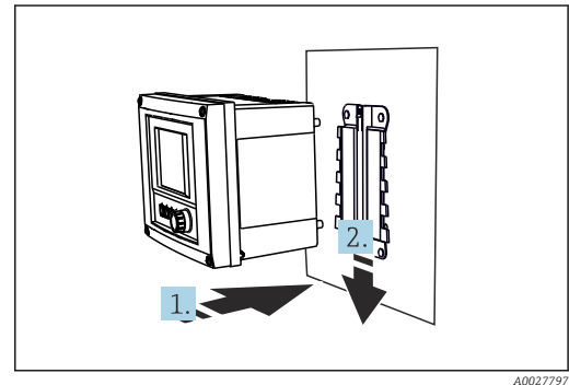
19 Sujete bien el equipo en el lugar deseado y fíjelo hasta oír el clic
