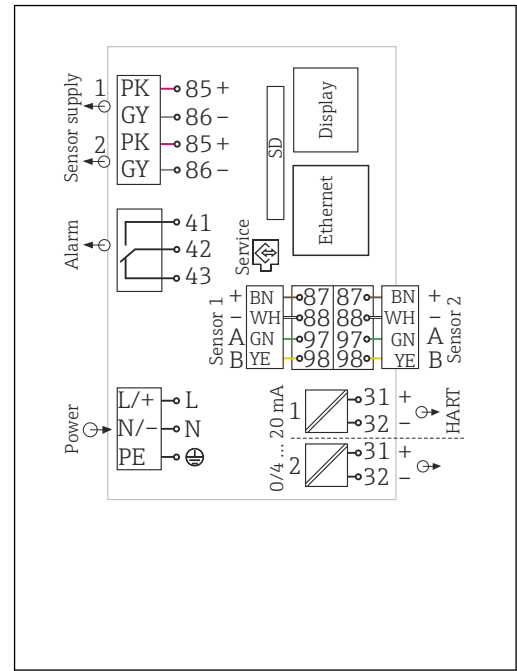
30 Diagrama de conexión completo con el ejemplo del BASE2-H o -L
