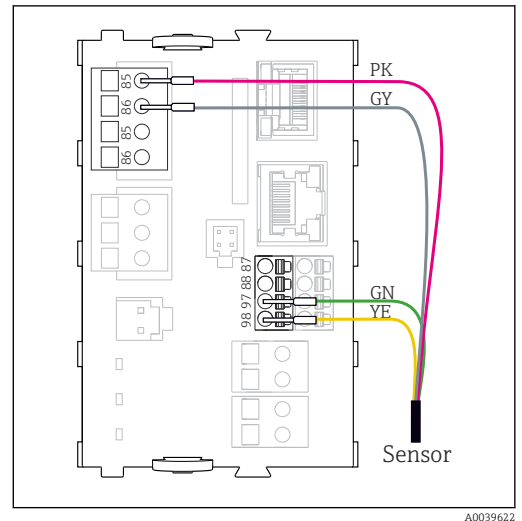
36 sensores con fuente de alimentación adicional
