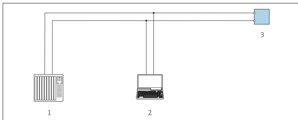
図 22 Modbus-RS485 プロトコル経由のリモート操作オプション (アクティブ)
