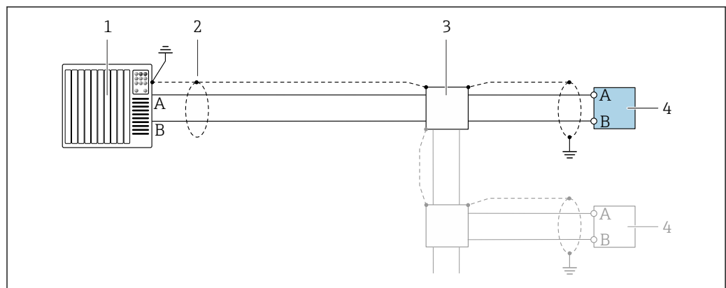
図 8 Modbus RS485 (非危険場所および Zone 2/Div. 2 用) の接続例
