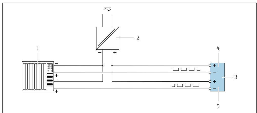
図 14 ダブルパルス出力（パッシブ）の接続例
