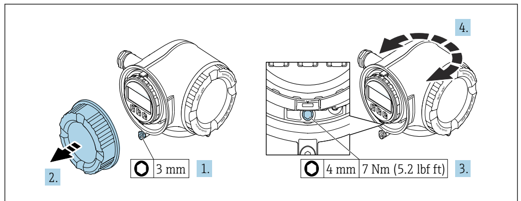
図5 非防爆ハウジング
