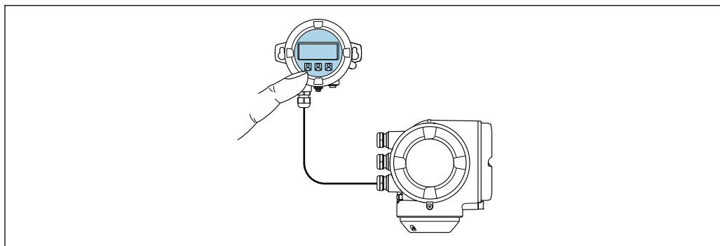
図 38 分離型ディスプレイと操作モジュール DKX001 を介した操作
