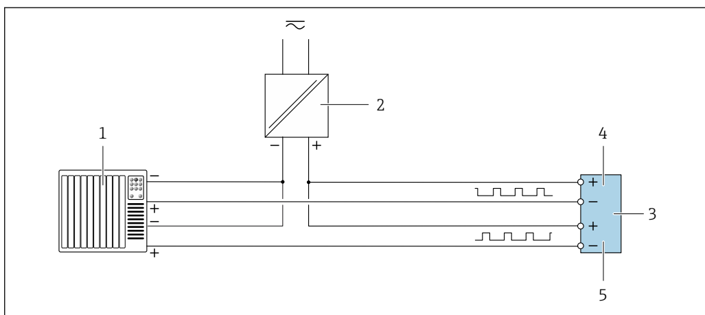
14 Пример подключения двойного импульсного выхода (пассивного)
