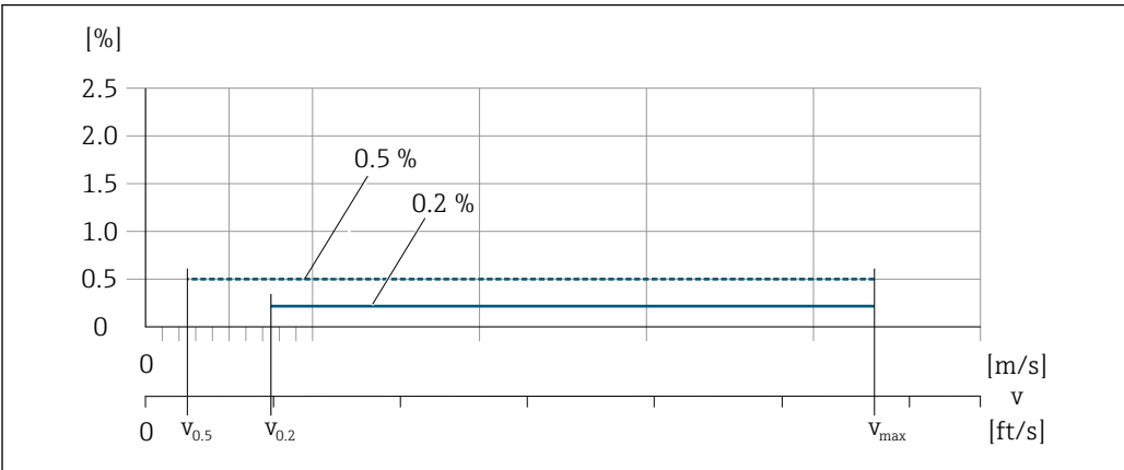
31 Линейная погрешность во всем диапазоне в % ИЗМ
