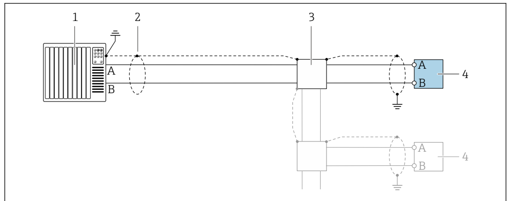
8 Пример подключения для интерфейса Modbus RS485, в невзрывоопасной зоне или зоне 2/разд. 2
