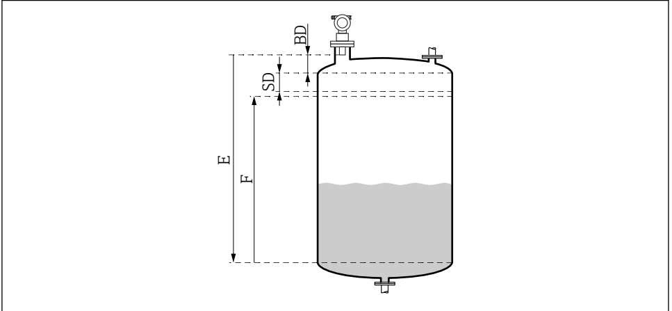
10 Parametry pracy przyrządu
