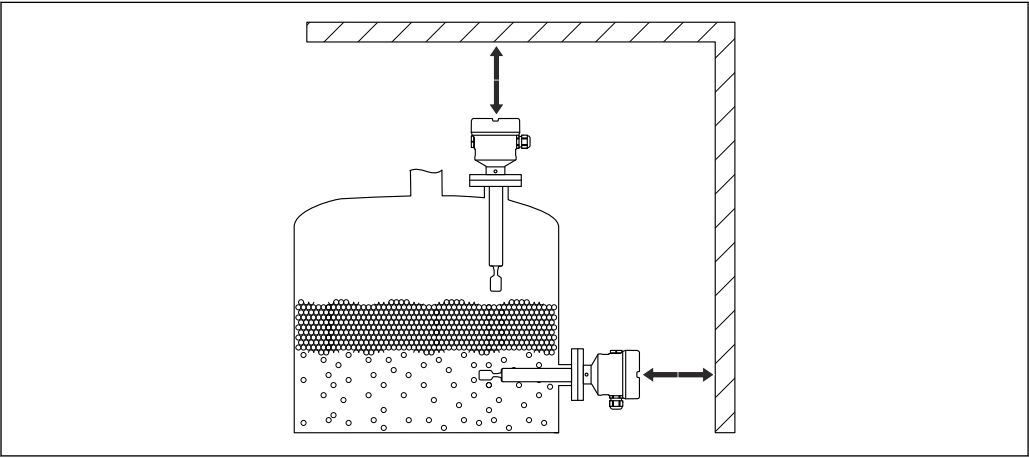
14 预留安装间隙
