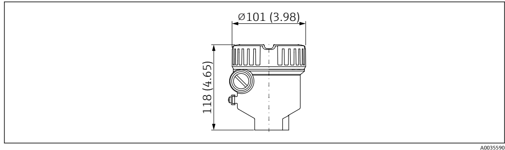
图 25 单腔体；铝，带涂层；适用于 Ex d/XP 防爆场合
