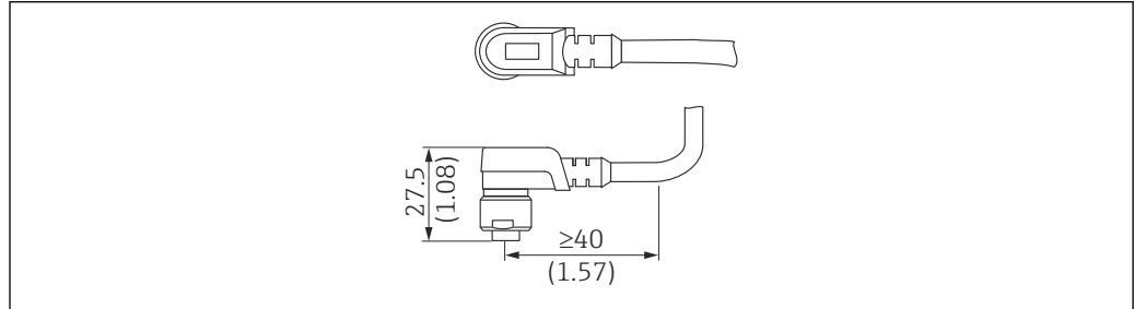
45 M12 插头, IP67 防护等级。测量单位 mm (in)
