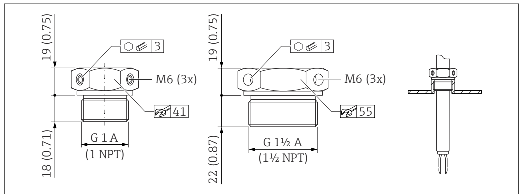
46 常压滑动套管 p_e = 0 bar (0 psi)。测量单位 mm (in)
