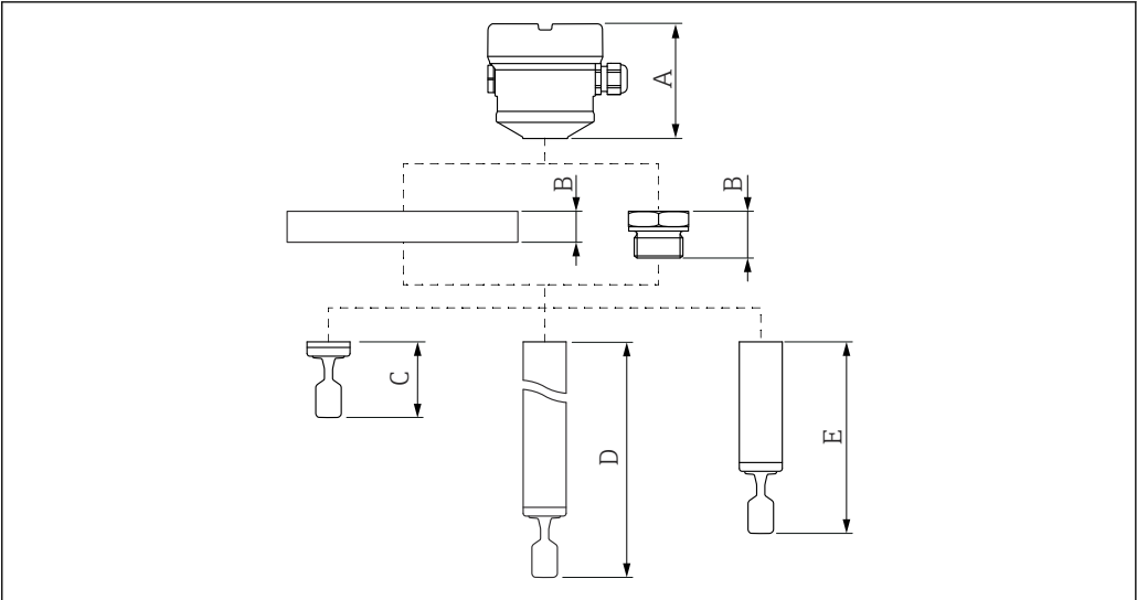
图 22 计算设备高度所需考虑的部件
