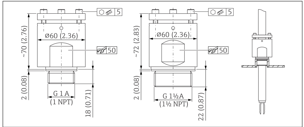
47 高压滑动套管。测量单位 mm (in)
