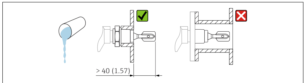
12 安装实例：测量高粘度液体。测量单位 mm (in)
