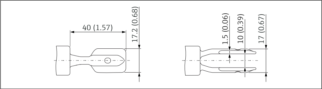
28 叉体。测量单位 mm (in)
