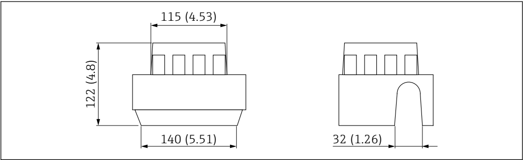
43 保护盖，适用单腔室铝外壳或 316L 外壳。测量单位 mm (in)
