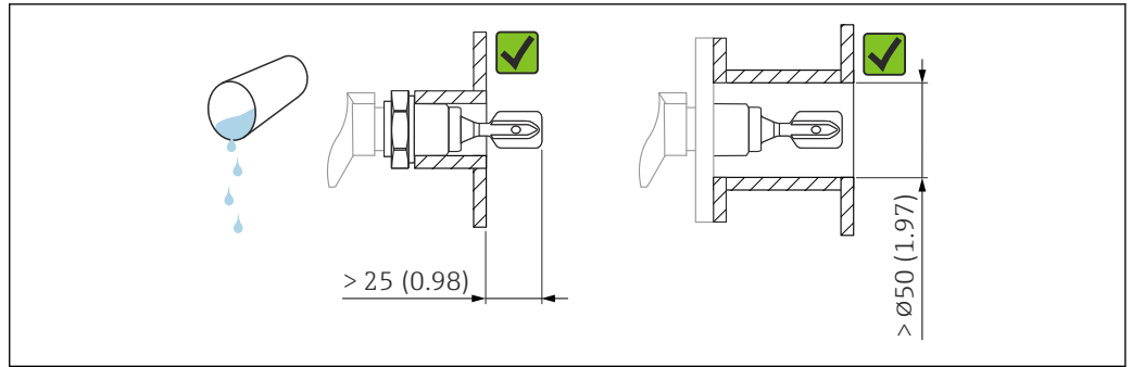
11 安装实例：测量低粘度液体。测量单位 mm (in)
