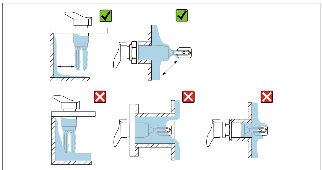
13 安装实例：测量高粘度过程介质
