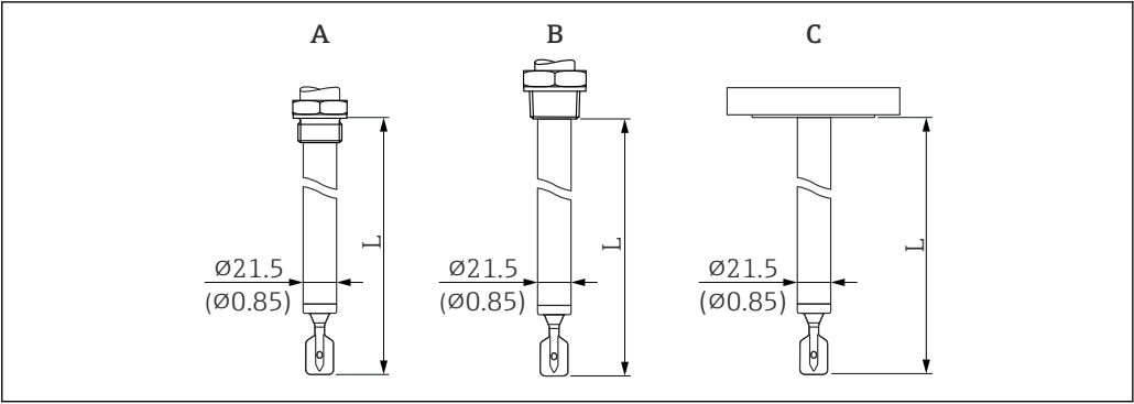
27 探头类型：延长管型、短管型；传感器长度 L
