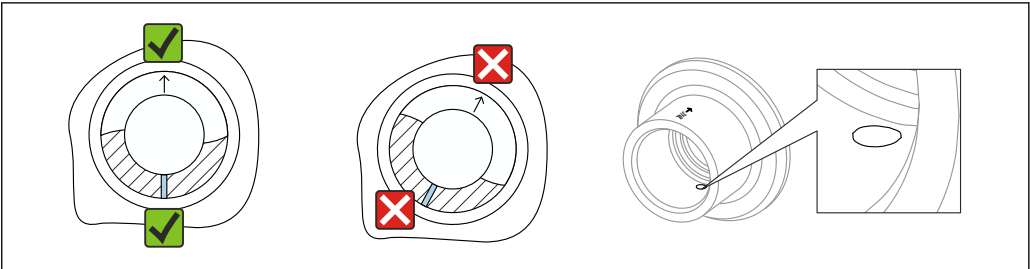
19 焊座，带泄漏检测孔
