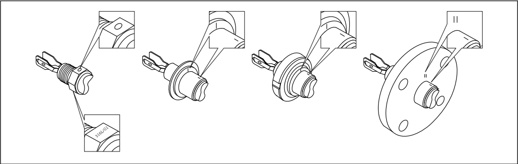
15 音叉安装位置标记
