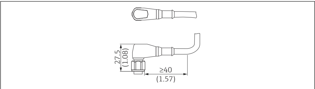
44 M12 插头，IP69 防护等级。测量单位 mm (in)
