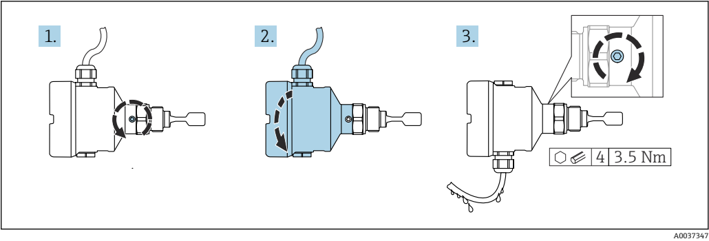
17 外壳带外部锁紧螺丝和排水回路
