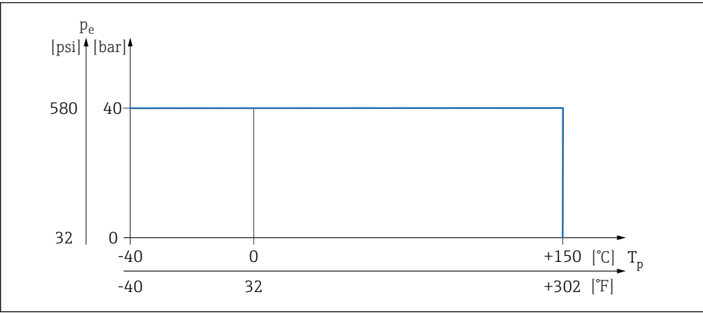
图 21 FTL41 的过程温度
