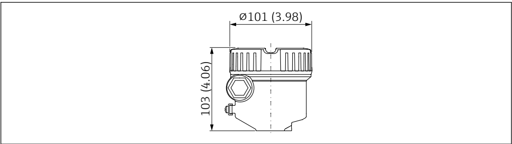
图 24 单腔体；铝，带涂层
