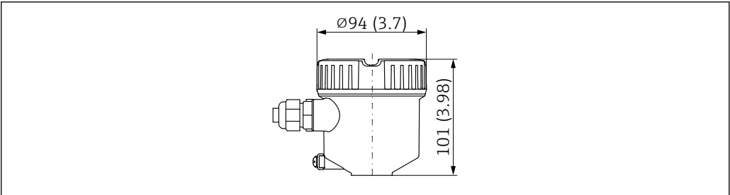
图 23 单腔体；塑料外壳
