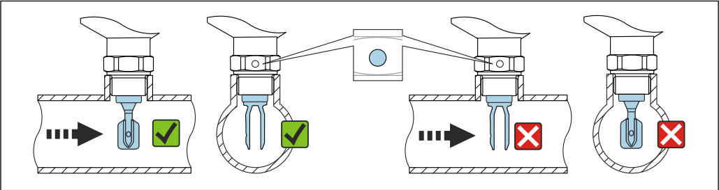
16 安装在管道中（注意叉体安装位置和标记）
