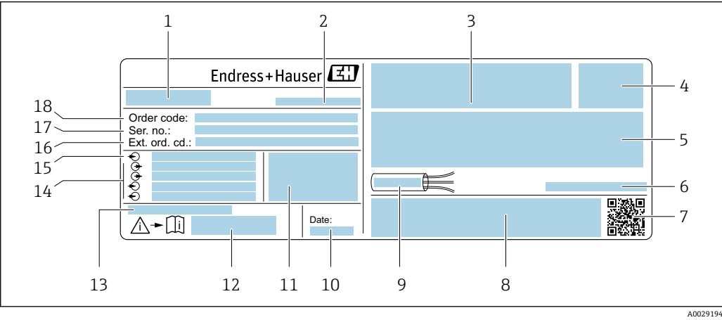
图 1 变送器的铭牌示意图
