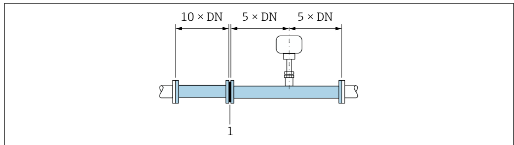
图 11 使用流量调节器时的推荐前后直管段长度
