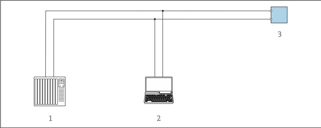
图 32 通过 Modbus-RS485 通信进行远程操作(有源信号)
