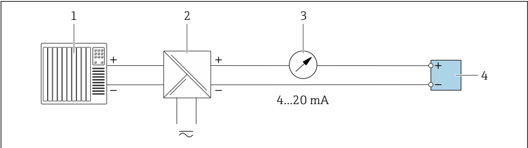
22 4...20 mA 电流输出（无源）的连接示例
