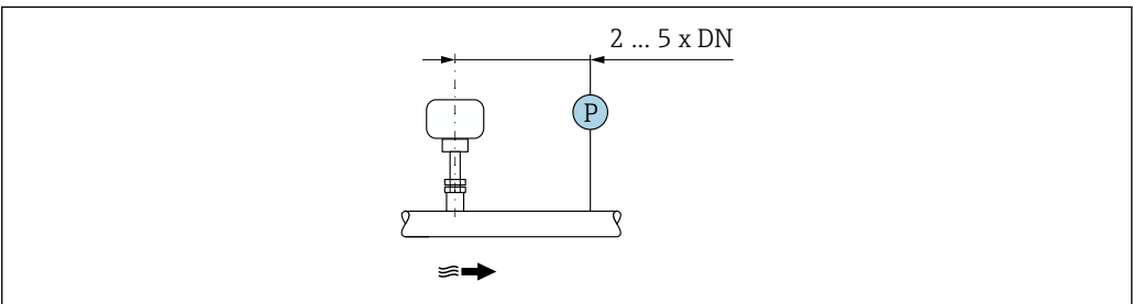
图 13 压力测量点的安装示意图 (P = 压力变送器)
