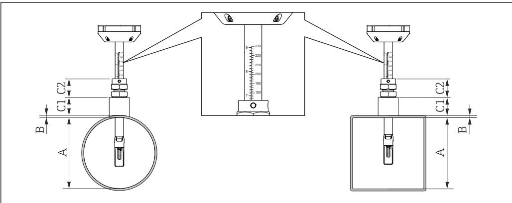
图 3 确定尺寸 A、B、C1 和 C2
