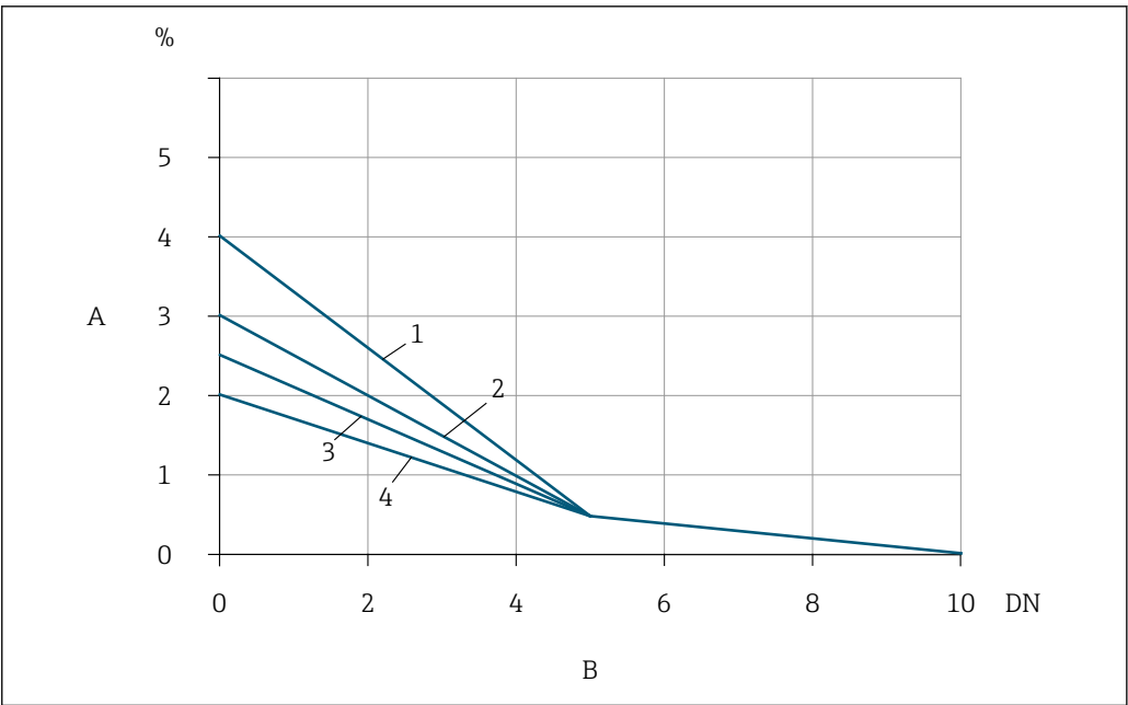
图 12 已安装流量调节器时可能存在的附加测量误差，与干扰因素和前管段类型相关
