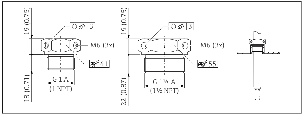
58 Manchons coulissants pour un fonctionnement sans pression p_e = 0 bar (0 psi). Unité de mesure mm (in)
