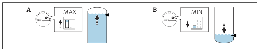
46 Position du commutateur sur l'électronique pour le mode de sécurité MAX/MIN
