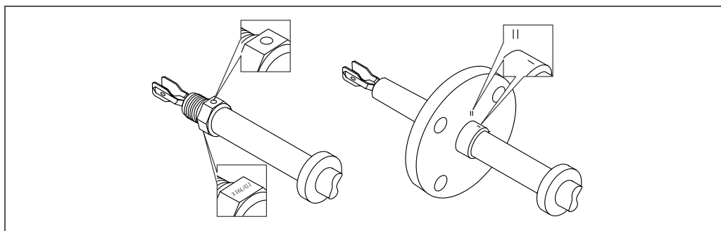
23 Repère pour l'alignement de la fourche vibrante
