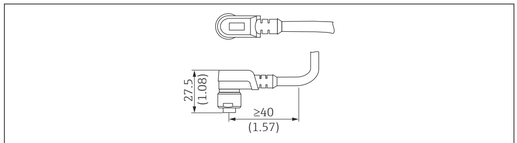
55 Connecteur femelle M12 IP67. Unité de mesure mm (in)
