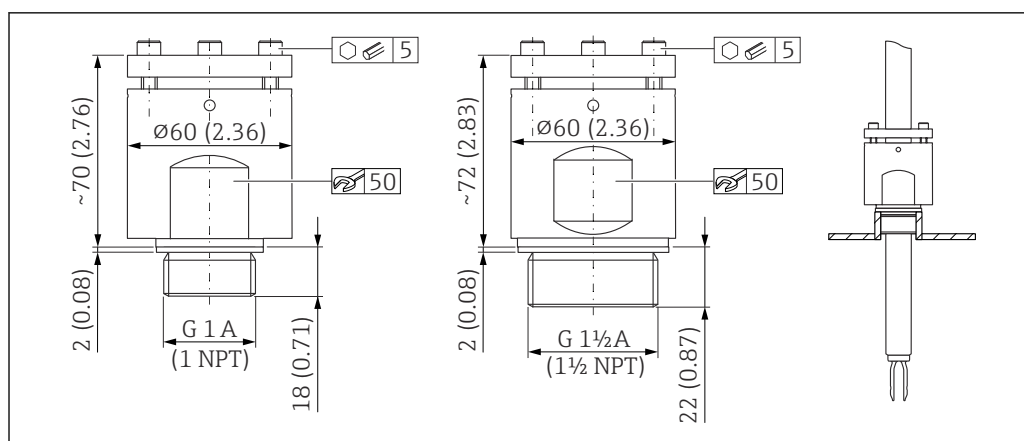
59 Manchons coulissants haute pression. Unité de mesure mm (in)
