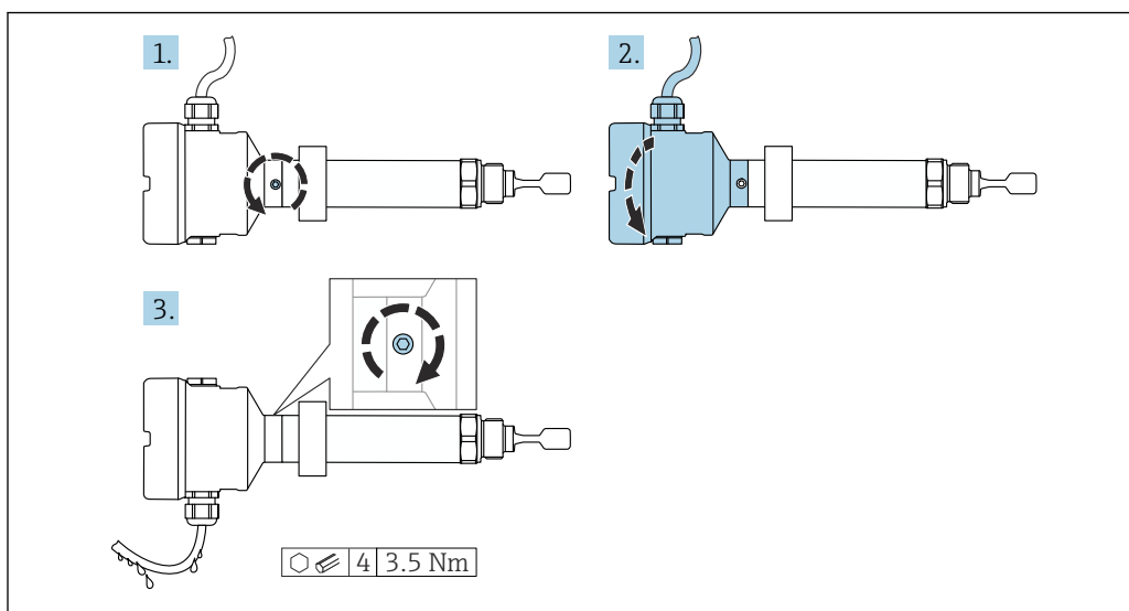
25 Boîtier avec vis de blocage externe et boucle de drainage
