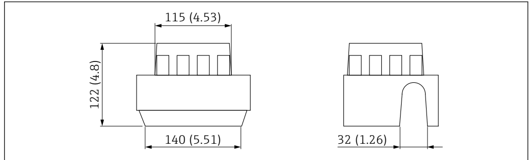
53 Capot de protection pour boîtier à compartiment unique, aluminium ou 316L. Unité de mesure mm (in)
