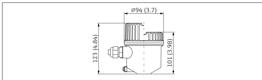
29 Compartiment unique ; boîtier plastique. Unité de mesure mm (in)
