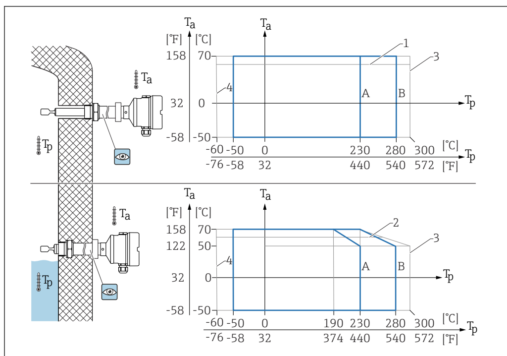
27 Température ambiante autorisée T_a au boîtier en fonction de la température de process T_p dans la cuve
