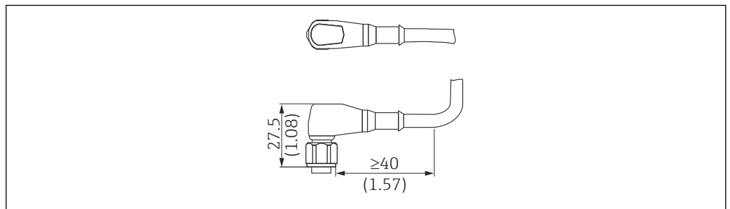
54 Connecteur femelle M12 IP69. Unité de mesure mm (in)
