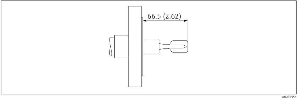
44 Exemple avec bride. Unité de mesure mm (in)
