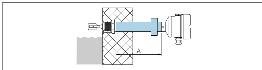
34 Réducteur thermique avec traversée en verre étanche aux gaz
