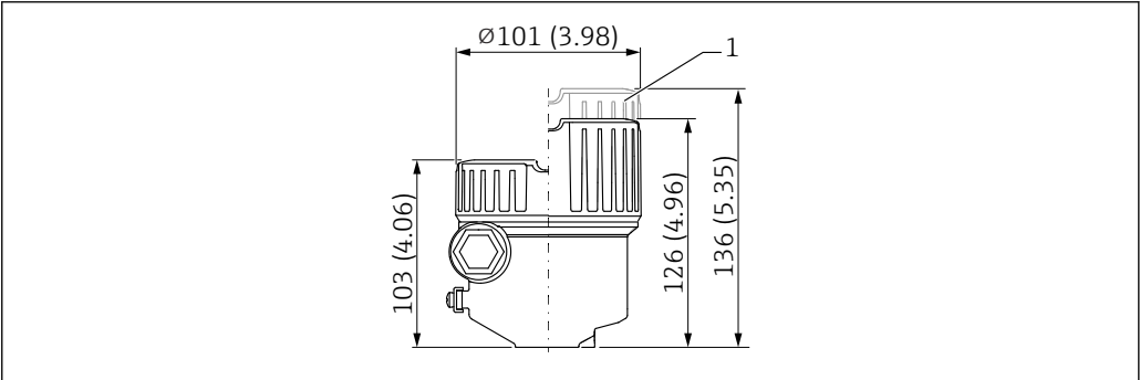
31 Compartiment unique ; aluminium, revêtu. Unité de mesure mm (in)
