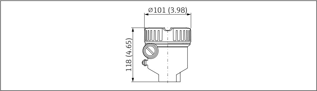
32 Compartiment unique ; 316L, fonte ; également avec agrément Ex d/XP. Unité de mesure mm (in)
