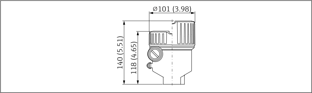
30 Compartiment unique ; aluminium, revêtu ; avec agrément Ex d/XP. Unité de mesure mm (in)
