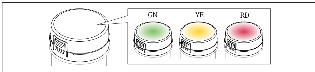
57 Module LED, la LED s'allume en vert (GN), jaune (YE) ou rouge (RD)
