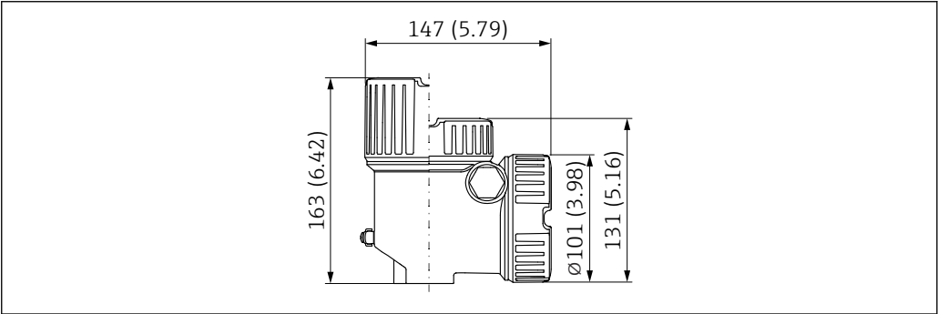
33 Compartiment double ; en L ; aluminium, revêtu ; également avec agrément Ex d/XP. Unité de mesure mm (in)
