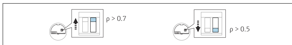
47 Position de commutation sur l'électronique pour la densité
