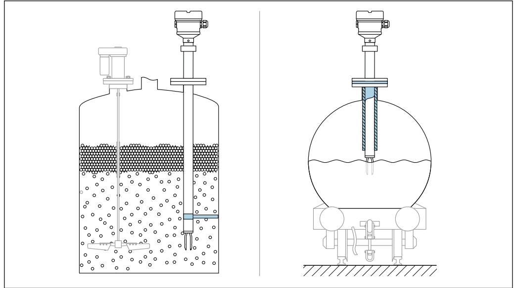
26 Exemples d'étayage en cas de charge dynamique
