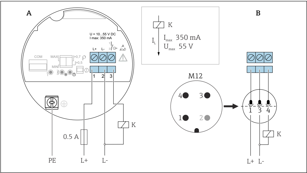
5 DC-PPN 3 fils, électronique FEL62 A Câble de raccordement avec bornes B Câble de raccordement avec connecteur M12 dans boîtier selon la norme EN61131-2
