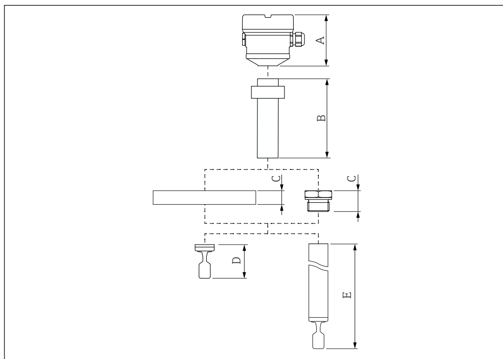
28 Composants permettant de déterminer la hauteur de l'appareil
