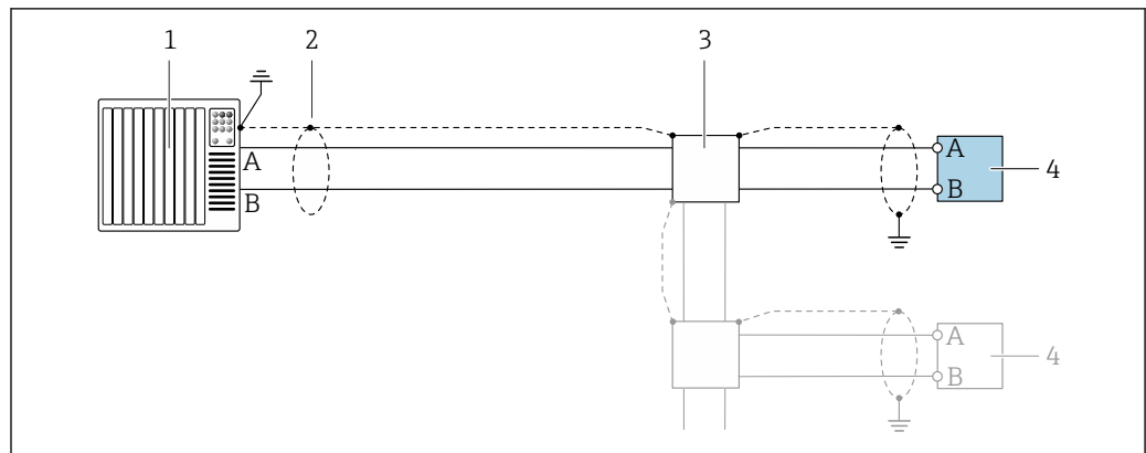
図 17 Modbus RS485 (非危険場所および Zone 2/Div. 2 用) の接続例
