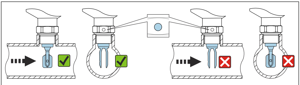
图 11 安装在管道中（考虑叉体安装位置和标记）
