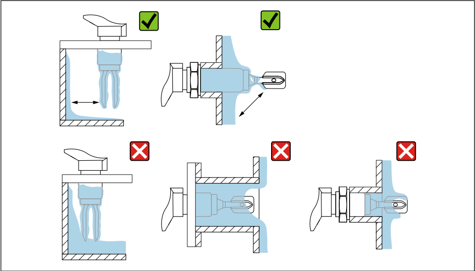
6 安装实例：测量高粘度过程介质
