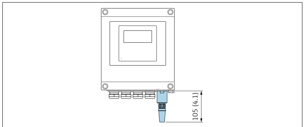
57 単位 mm (in)
