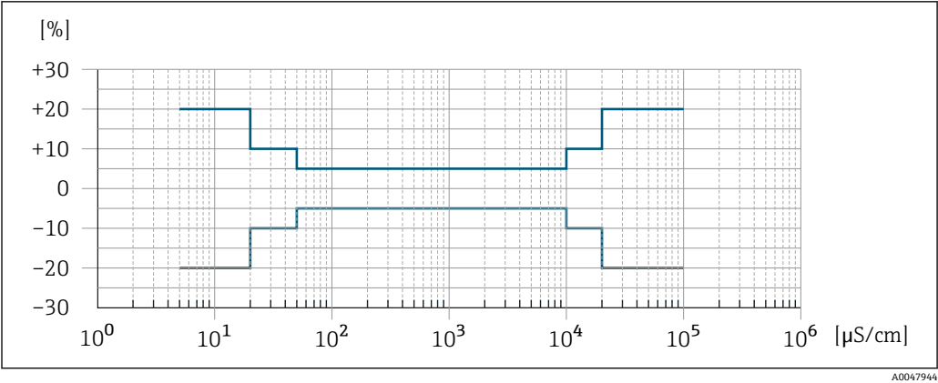
図 25 測定誤差（オプション：「校正された導電率測定」のオーダーコード、オプション CW）
