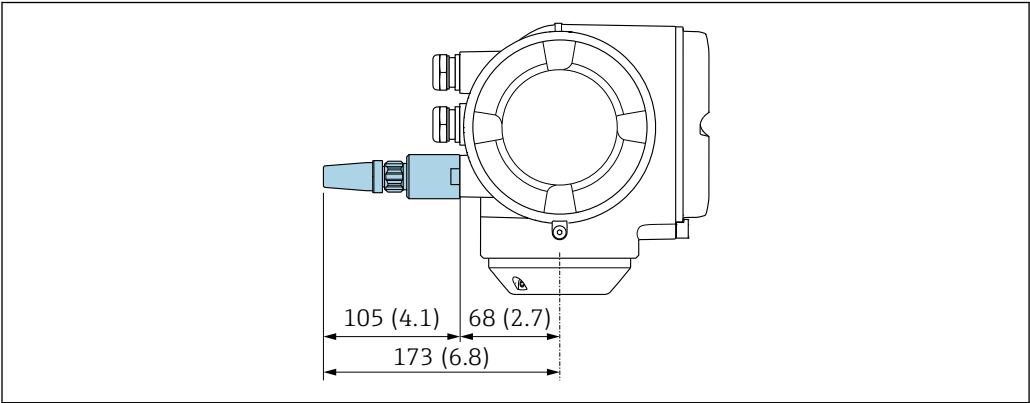
図 59 単位 mm (in)
