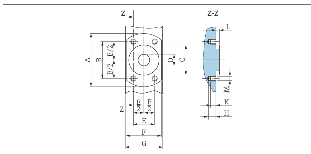
51 プロセス接続なしの正面図
