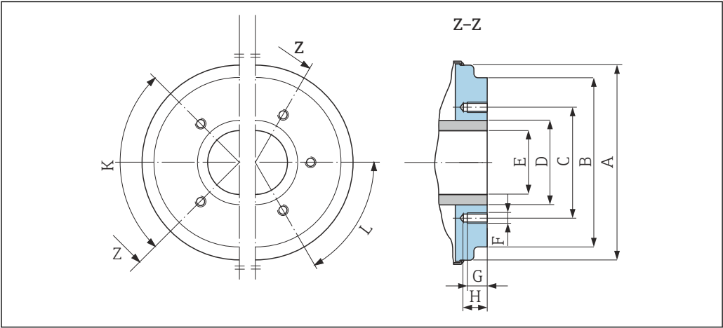
図 62 プロセス接続なしの正面図
