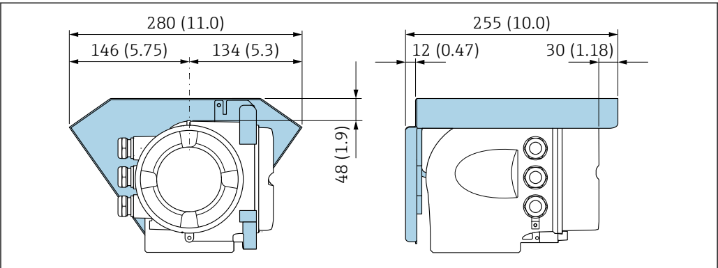
図 32 Proline 500 用の日除けカバー、単位 mm (in)
