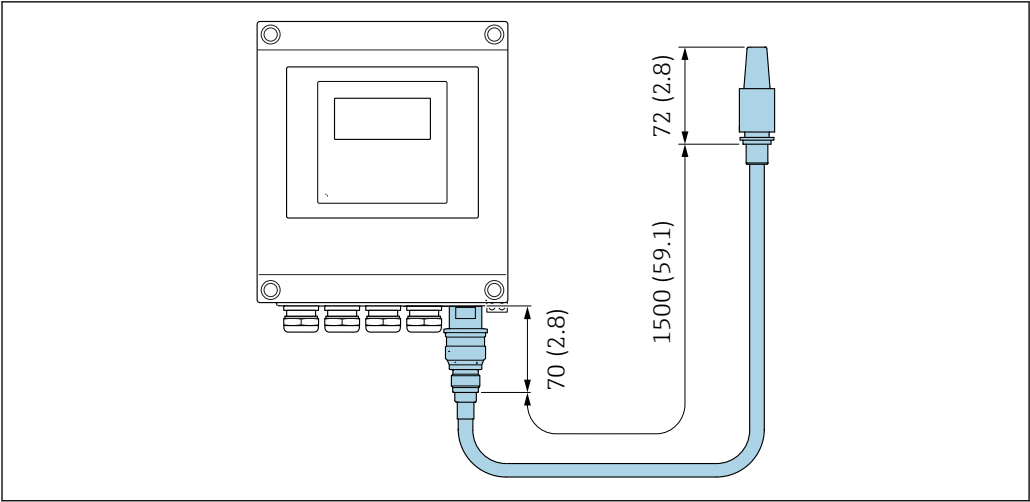
図 66 単位 mm (in)
