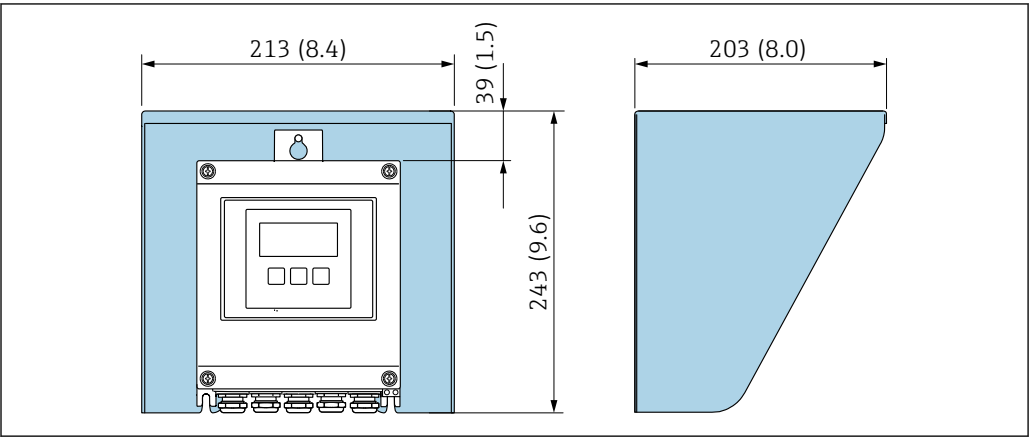
図 31 Proline 500 – デジタル用の日除けカバー、単位 mm (in)
