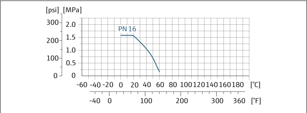
38 プロセス接続材質：PVC-U
