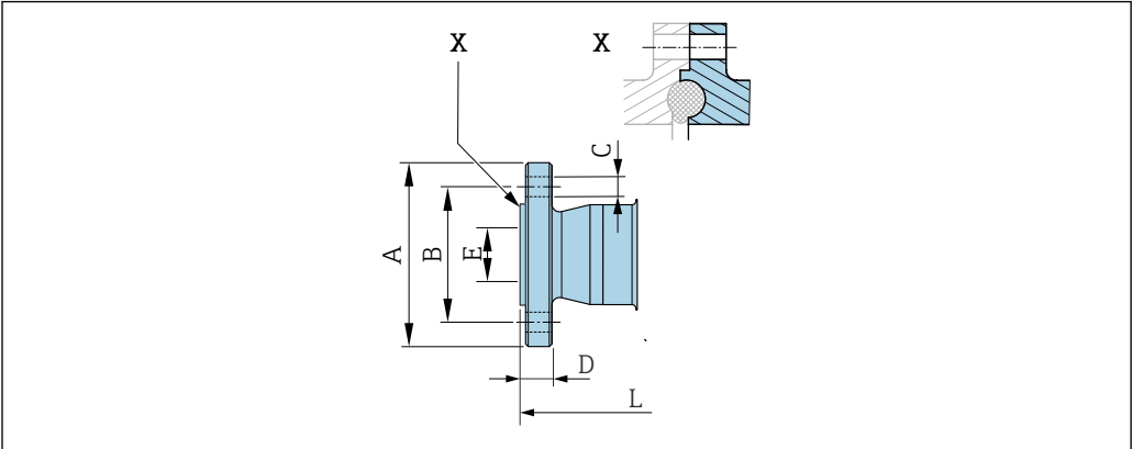
図 53 Xの詳細：非対称型プロセス接続；着色部分が供給されます。
