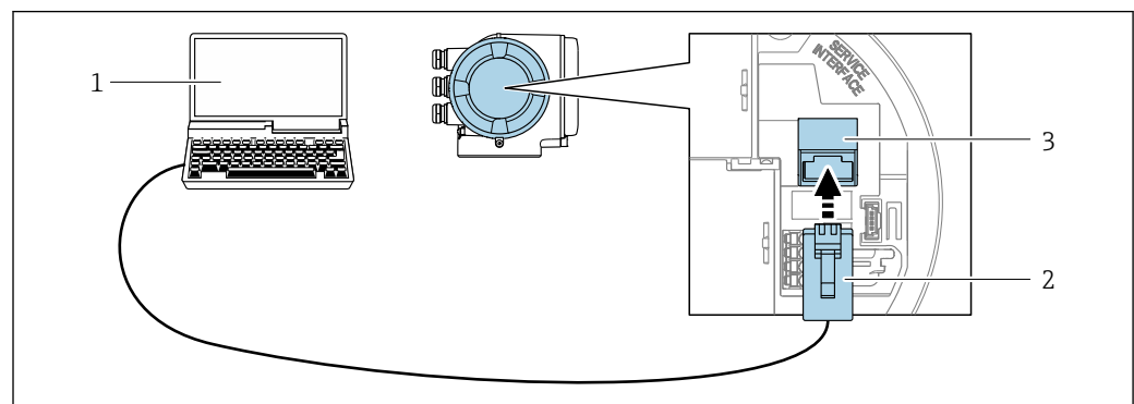
図 84 サービスインターフェイス (CDI-RJ45) 経由の接続
