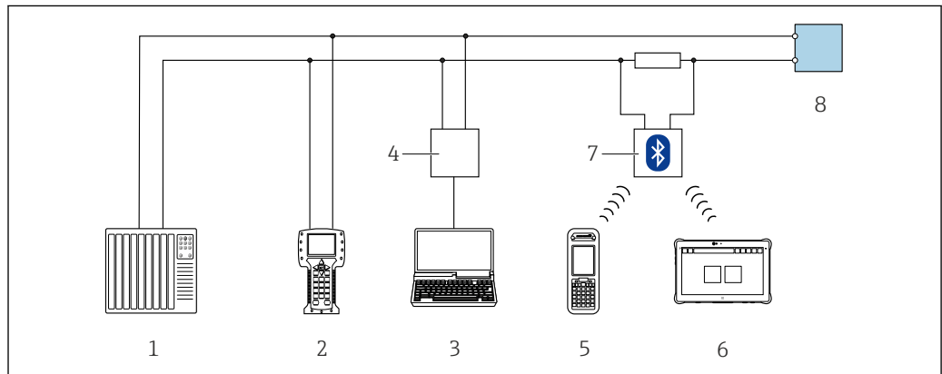
図 72 HART プロトコル経由のリモート操作オプション（アクティブ）
