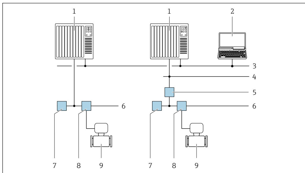
図 74 FOUNDATION フィールドバスネットワークを介したリモート操作用のオプション
