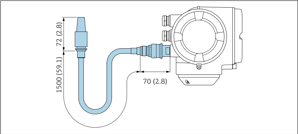
図 60 単位 mm (in)
