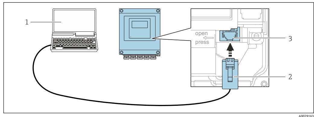
図 83 サービスインターフェイス (CDI-RJ45) 経由の接続
