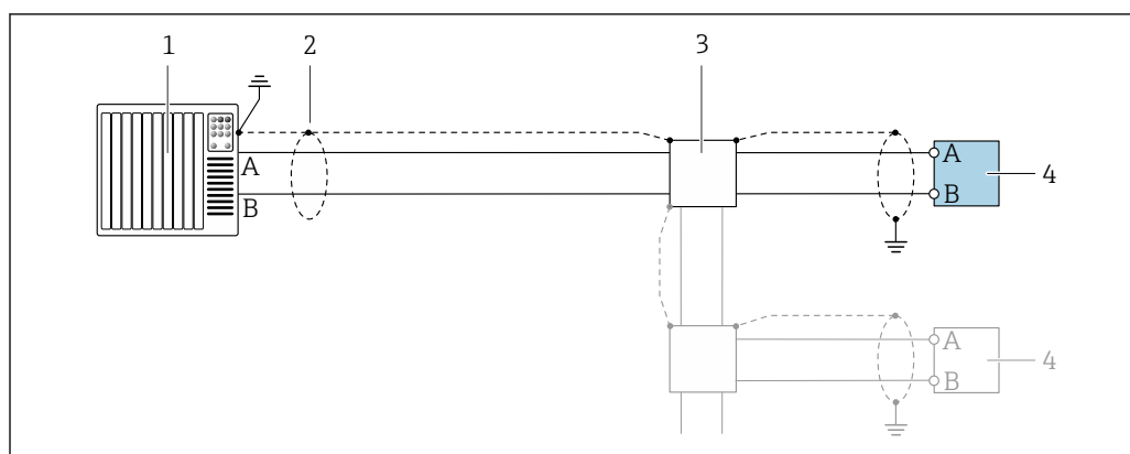
図 12 Modbus RS485（非危険場所および Zone 2/Div. 2 用）の接続例
