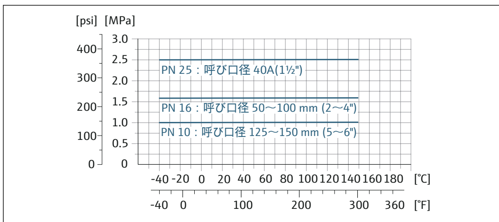
図 49 プロセス接続材質 : ステンレス 1.4404 (SUS F316L 相当)
