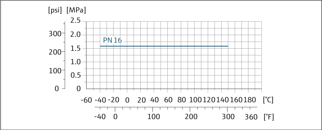
44 プロセス接続材質：ステンレス 1.4404 (SUS F316L 相当)
