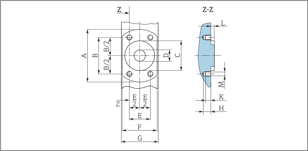
図 61 プロセス接続なしの正面図
