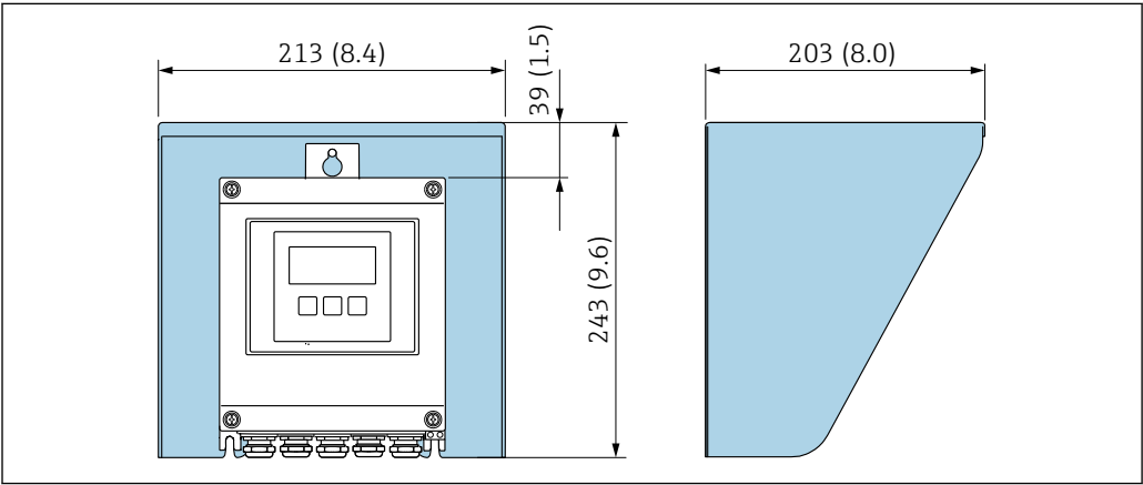
63 Proline 500 – デジタル用の日除けカバー、単位 mm (in)
