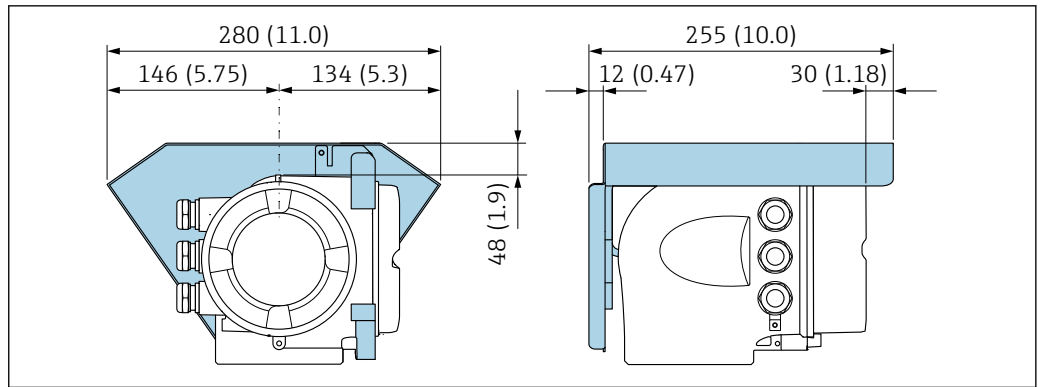
64 Proline 500 用の日除けカバー、単位 mm (in)
